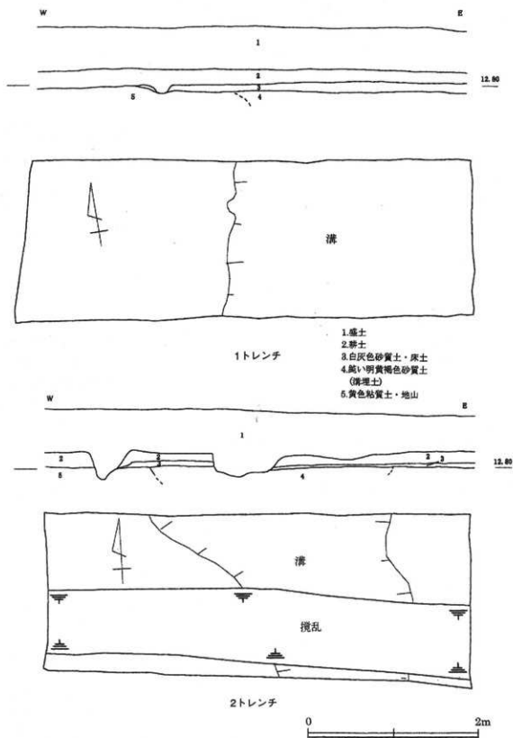
図20 遺構平面図・土層断面図
