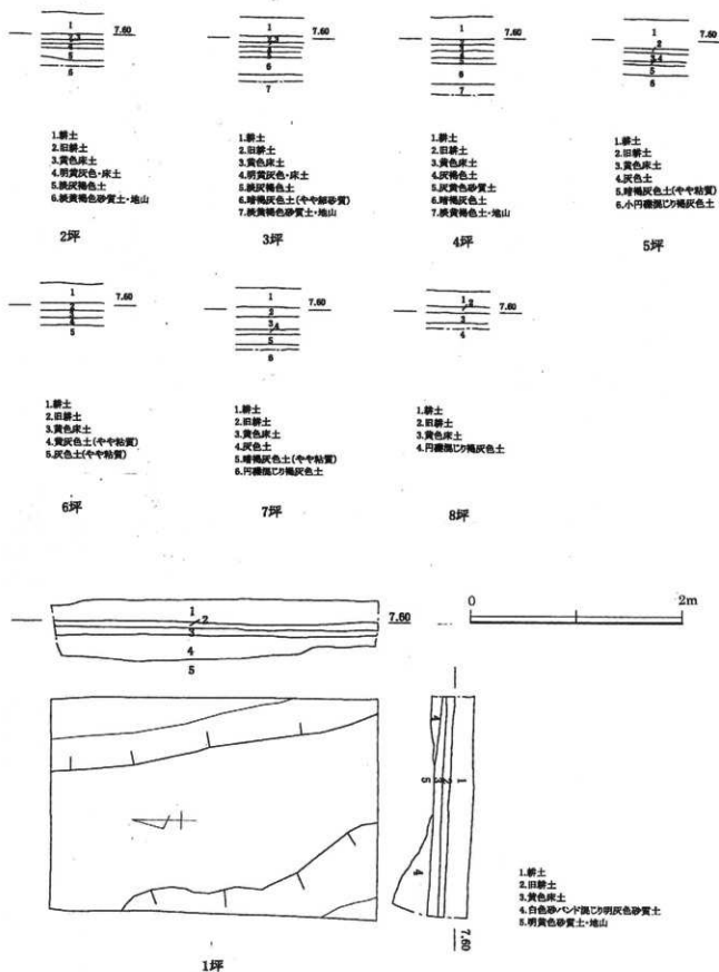
図31 平面・土層断面図
