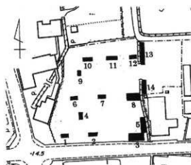
図108 トレンチ配置図(1/2,500)
