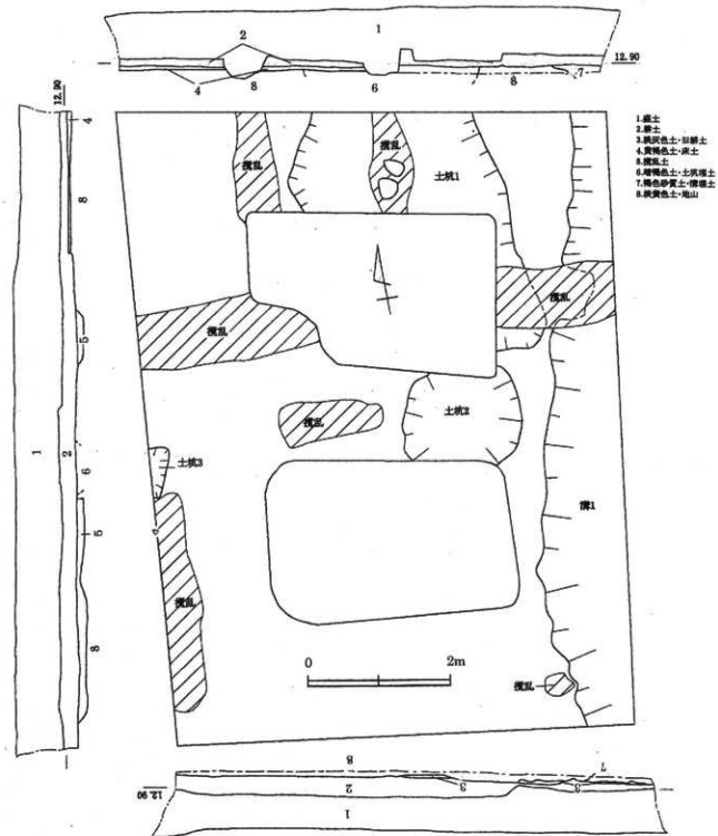
図34 遺構平面図・土層断面図
