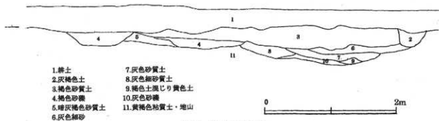
図24 溝土層断面図
