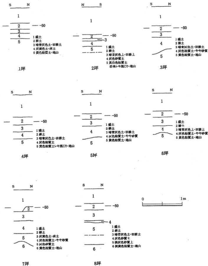
図90 土層断面図
