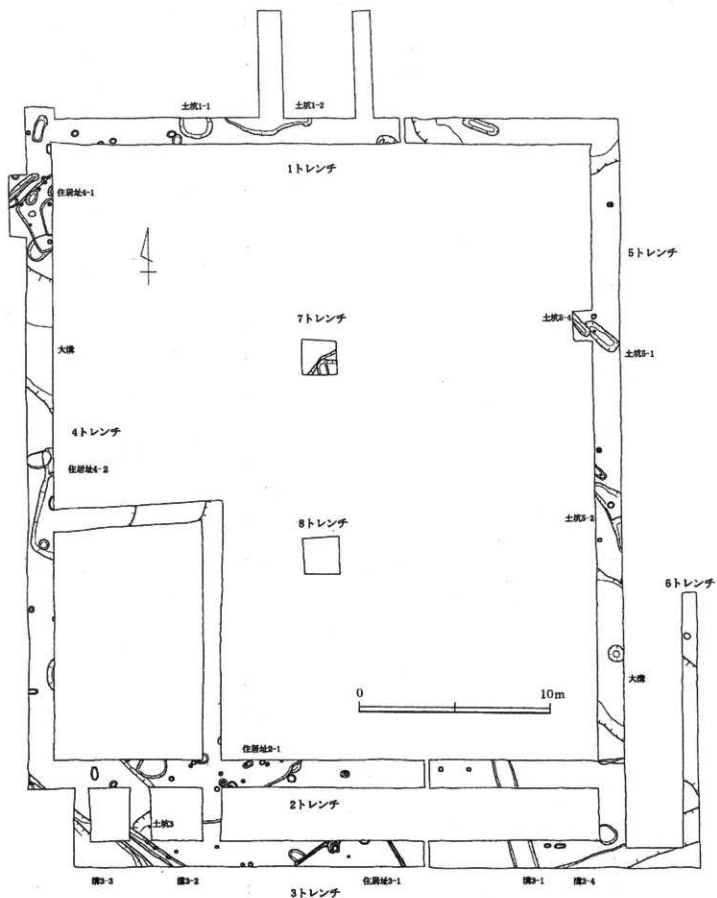
図54 遺構配置図
