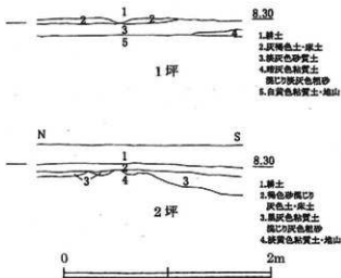
図126 土層断面図
