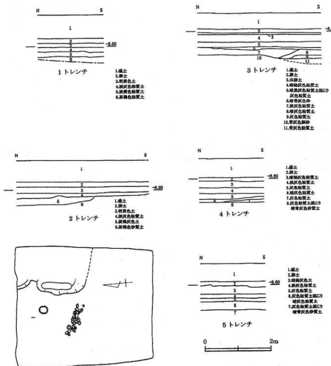
図98 遺構平面図・土層断面図
