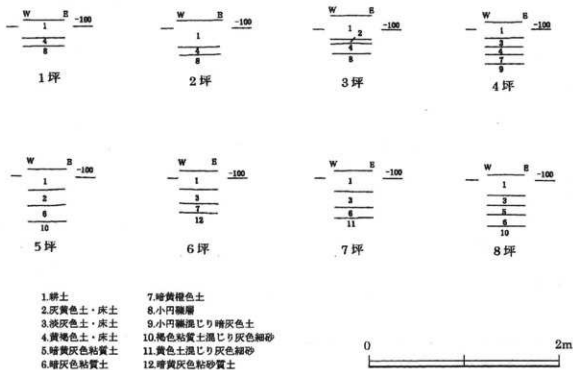
図28 土層断面図
