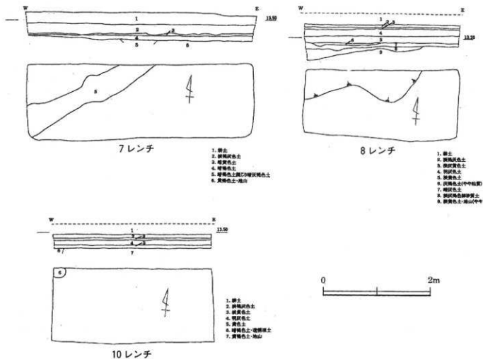
図43 遺構平面図・土層断面図(2)
