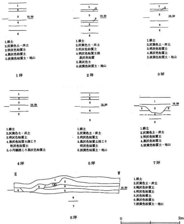
図71 土層断面図(1)
