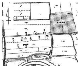
図35 トレンチ配置図（1/2,500）
