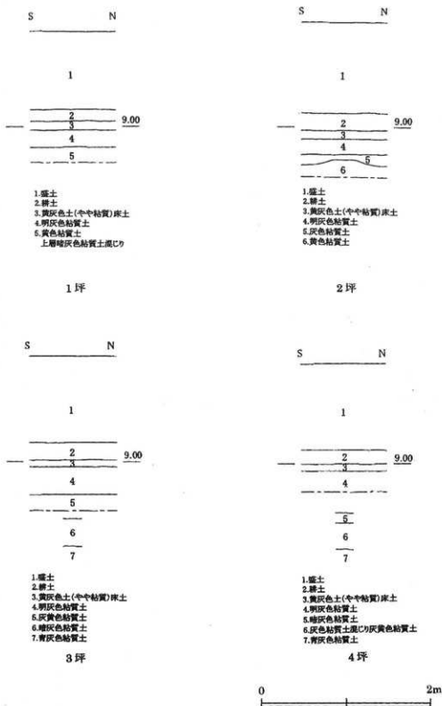
図69 土層断面図
