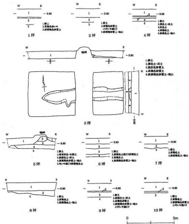
図95 遺構平面図・土層断面図
