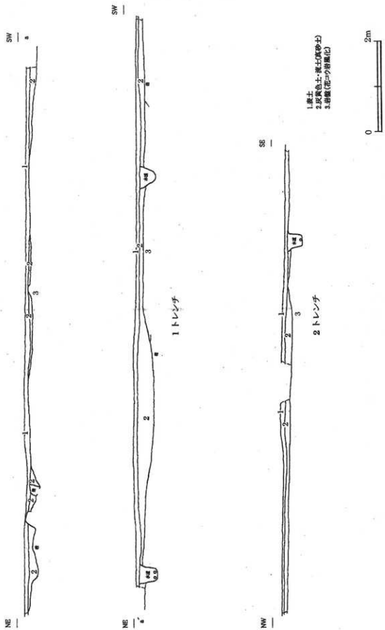
図81 土層断面図
