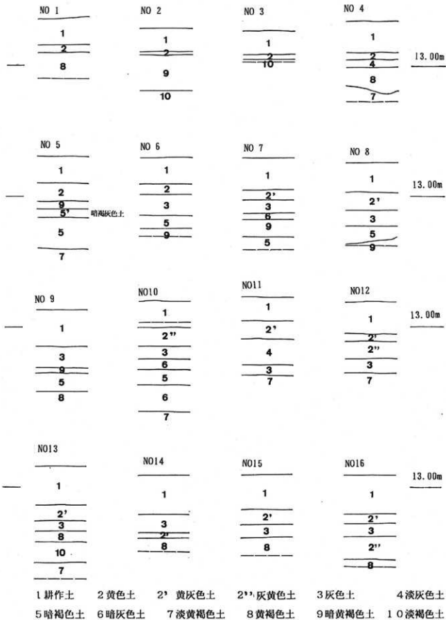
第3图 調査区土層断面图
