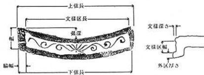
軒瓦各部位名称
