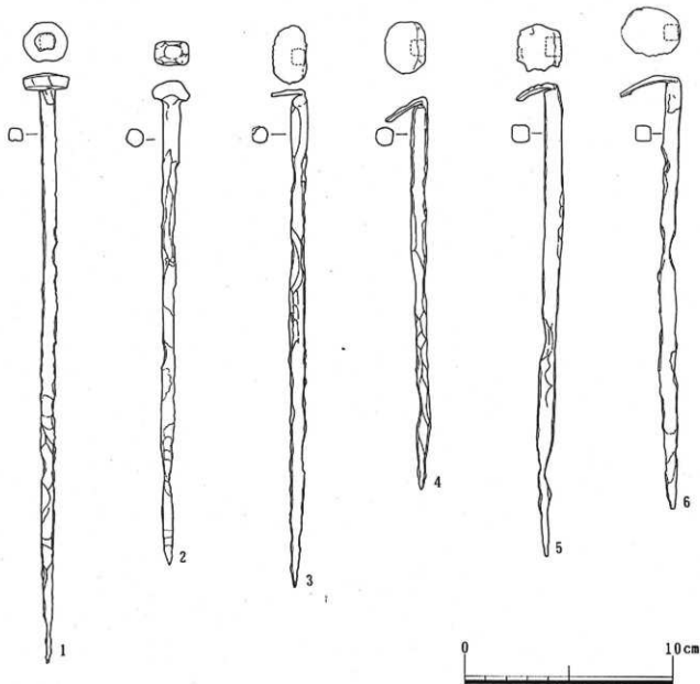
瓦釘実測図(1)
