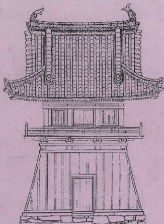
斑鳩寺鐘樓 (西立面図)
