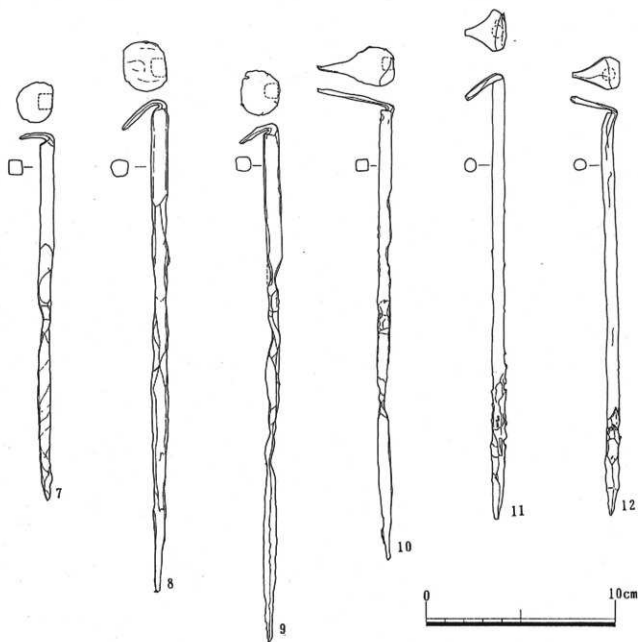
瓦釘実測図(2)
