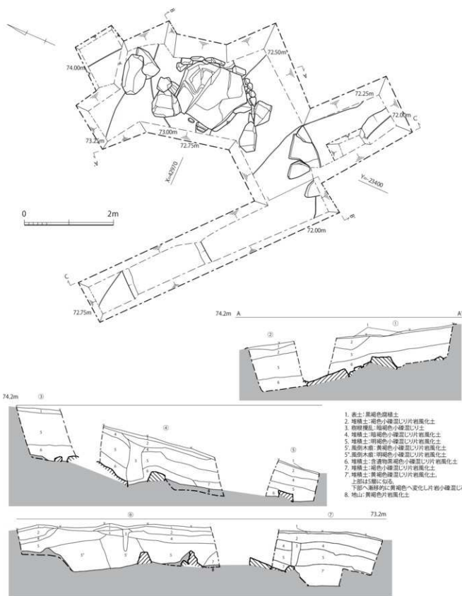
第7図 3・9号トレンチ平面図及び断面図 (1/60)
