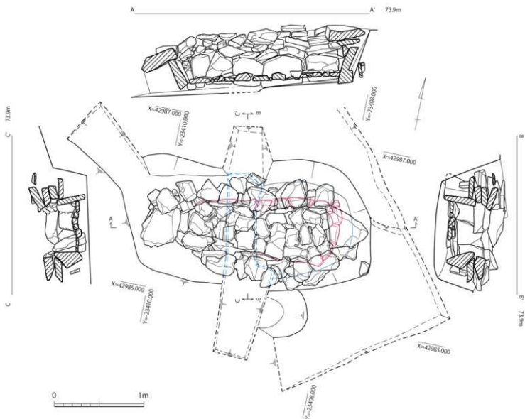
第5図 1号小石室実測図 (1/30)
