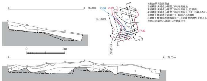
第6図 5号トレンチ土層断面図 (1/60)
