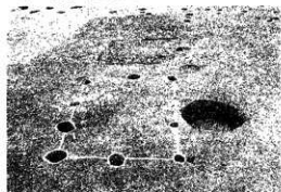
第3号掘立柱建物跡・第2号土坑
