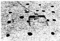
第19・20号掘立柱建物跡・第38号土坑
