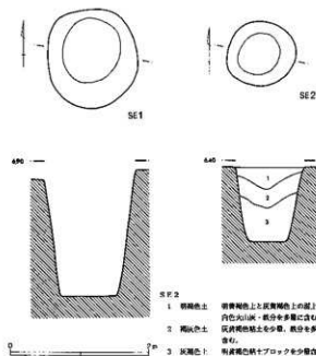
第42図 第1・2号井戸跡
