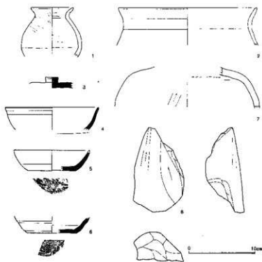
第43図 グリッド出土遺物
