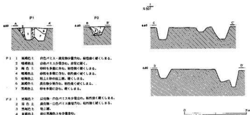
第18図 第1号掘立柱建物跡
