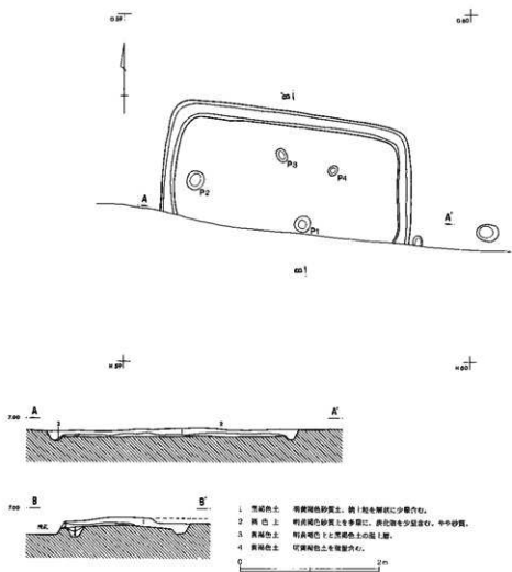
第15图 第3号住居跡
