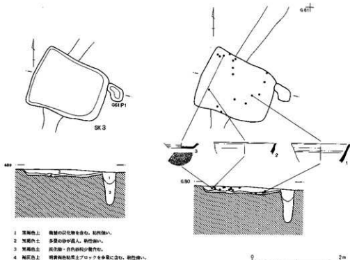
第20図 第3号土坑
