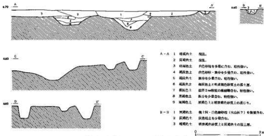
第40図 第6・7・9号溝跡(2)
