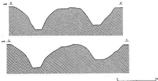
第38図 第4・5号溝跡(2)
