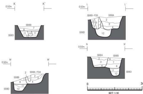
第21図 SB8 断面図(2)
