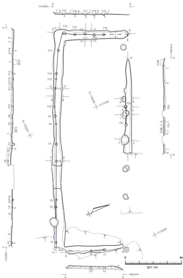
第90図 SB13B 平面断面図
