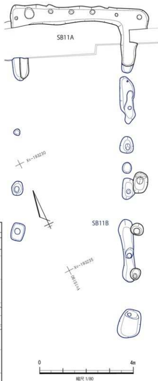
第65図 SB11A、11B 平面図
