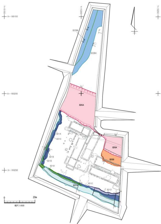
第105図 SD 1、SD 29、SD 5 平面図
