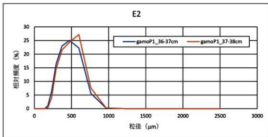
第181図 ジオスライザーNo.1(P1)のイベント砂層E2の粒度分布
