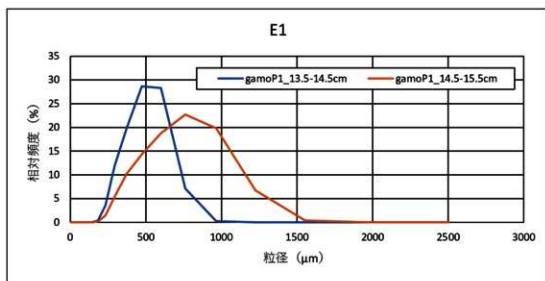
第180図 ジオスライサーNo.1(P1)のイベント性砂層E1の粒度分布
