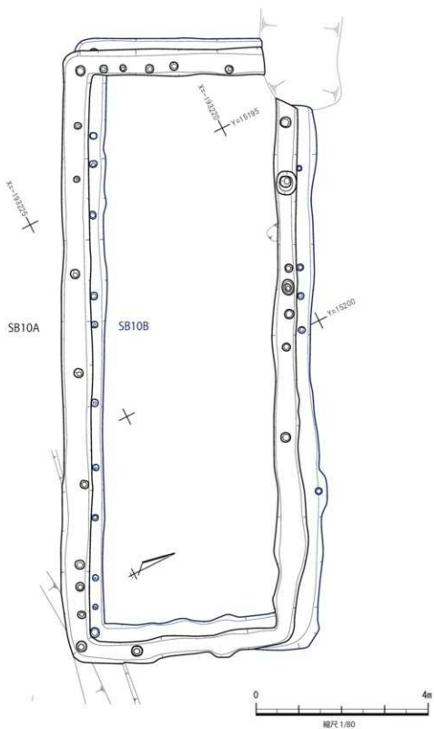
第34図 SB10A、10B 平面図
