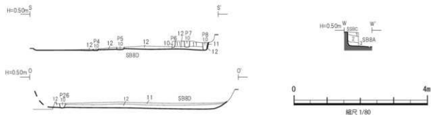
第27図 SB8C、8D 断面図
