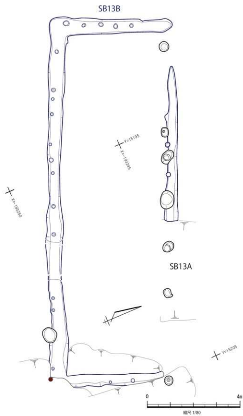
第77図 SB13A、13B 平面図
