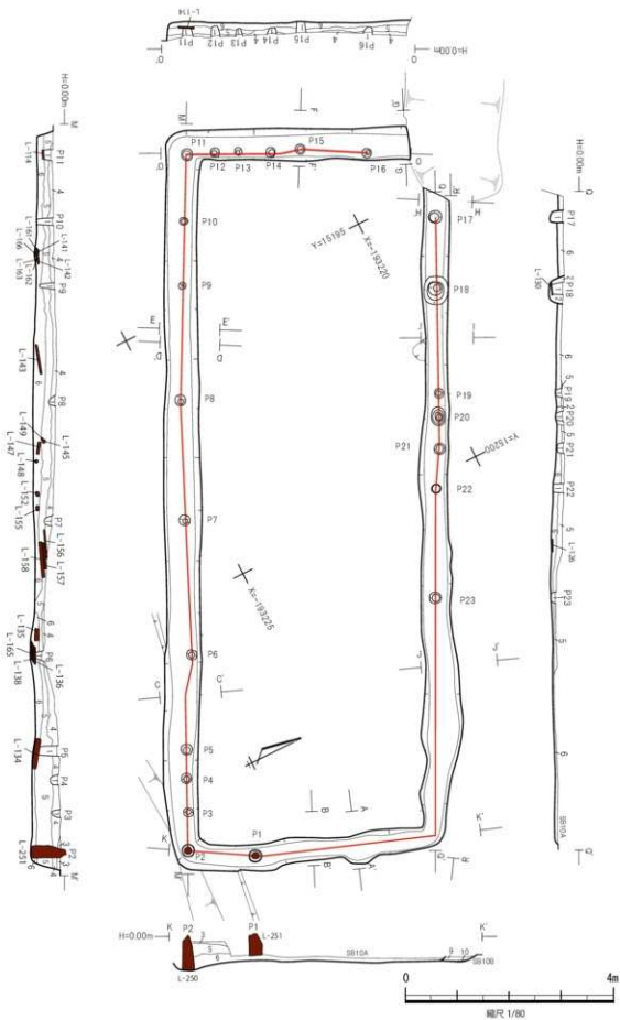
第35図 SB10A 平面断面図
