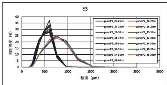
第182図 ジオスライザーNo.2(P2)のイベント砂層E3の粒度分布
