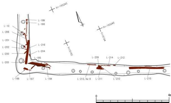
第91図 SB13B 遺物出土状況図
