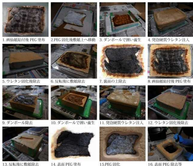
第 187 図 実験 3 PEG 含浸法処理工程
