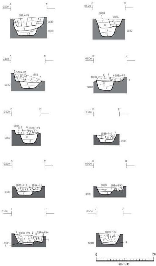
第20図 SB 8 断面図 (1)
