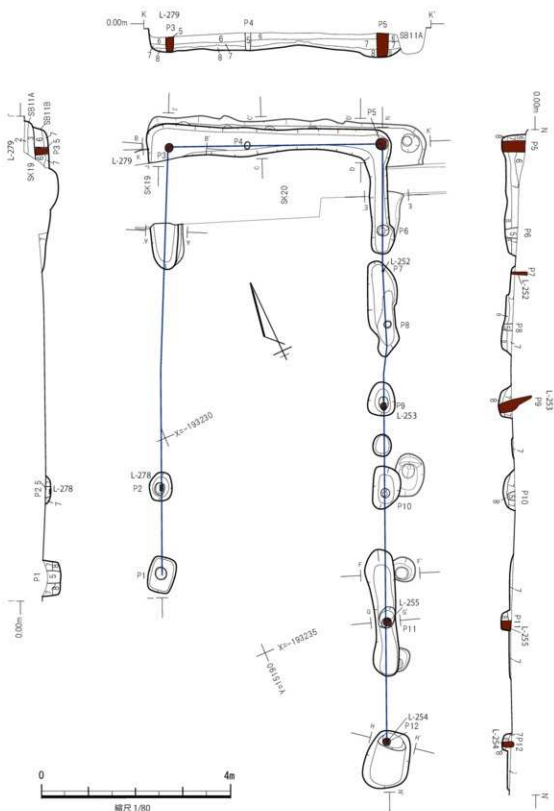
第67図 SB11B 平面断面図
