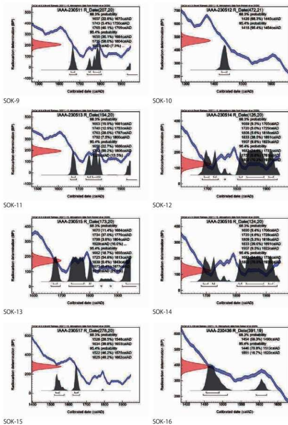
第167図 暦年較正年代グラフ(2)
