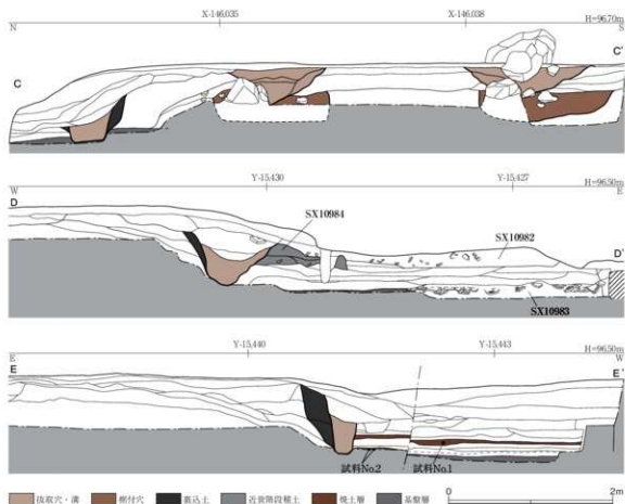
第12図 経蔵 (C区) 土層図 1 : 50
