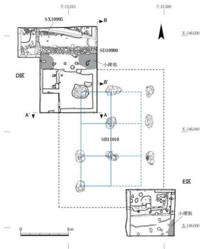
第19図 鐘樓調査区 (D・E区) 遺構平面図 1 : 200
