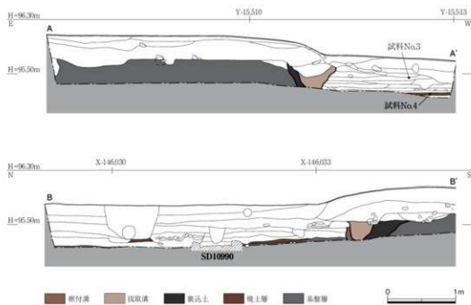
第20図 鐘樓調査区 (D区) 土層図 1 : 50
