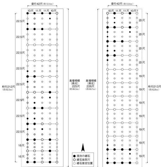
第31図 興福寺西室(左)・中室(右)柱配置復原模式図
