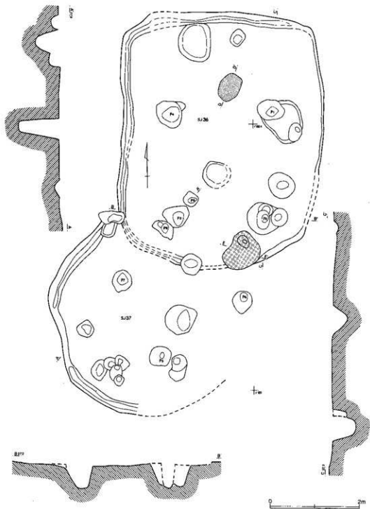
第362图 第36-37号住居跡(1)
