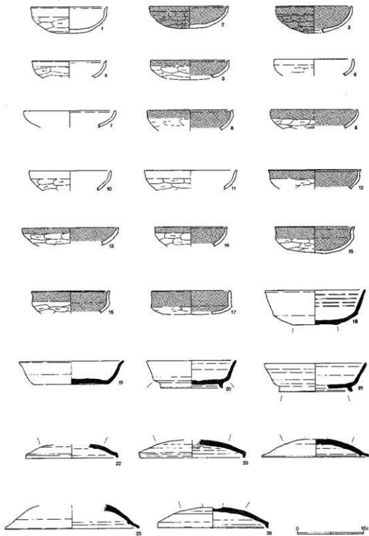
第353图 第5号住居跡出土遺物(7)
