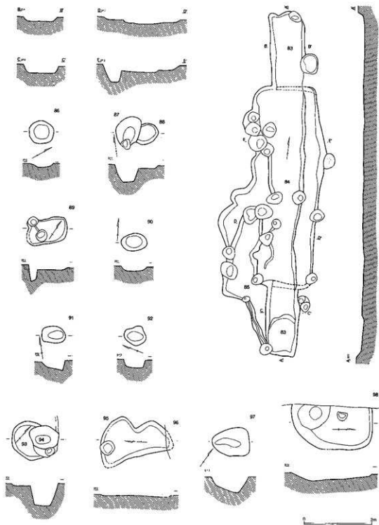
第451圖 土坑⑤
