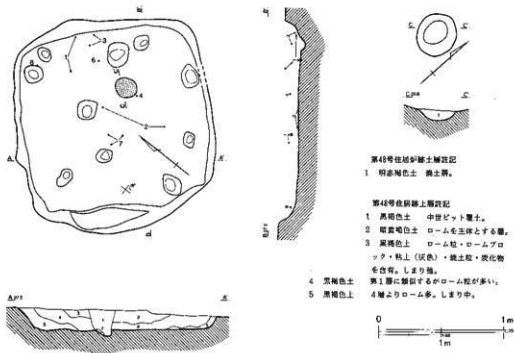
第394図 第48号住居跡
