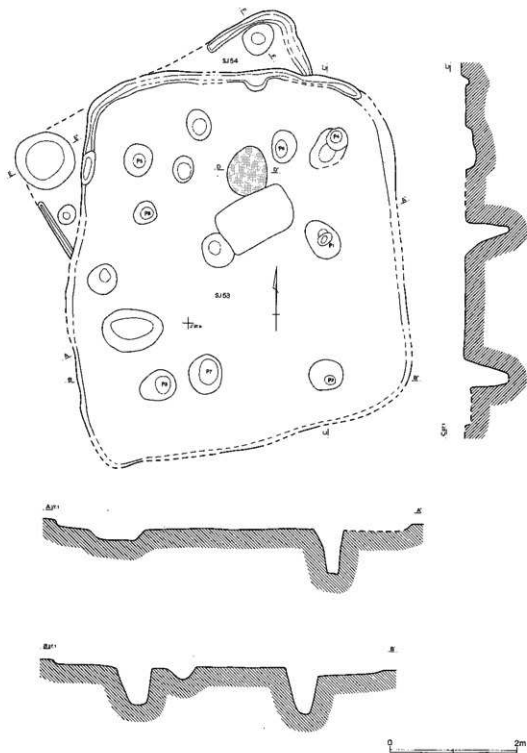
第402图 第53・54号住居跡(1)
