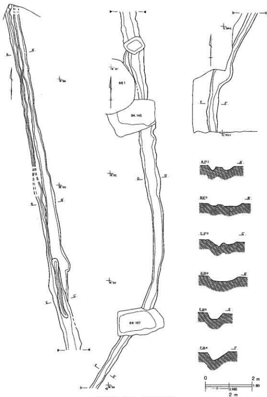
第481图 第1~4.6号清跡
