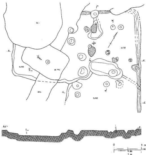
第439図 第59号住居跡
