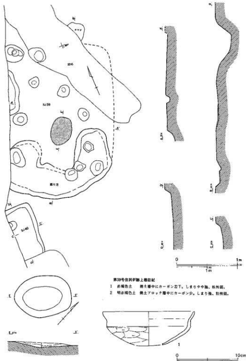
第386図 第39号住居跡、出土遺物
