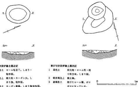
第383図 第36・37号住居跡②
