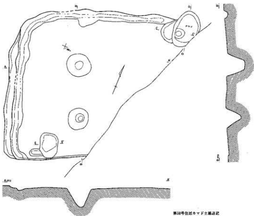
第38号住居カマド土層図記
