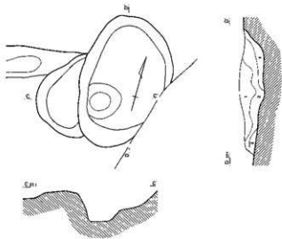
第438図 第38号住居跡
