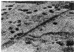
第4号溝
