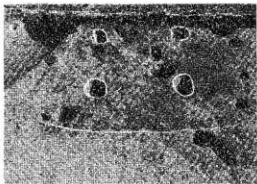
第29号住居跡
