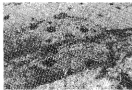
第51号住居跡
