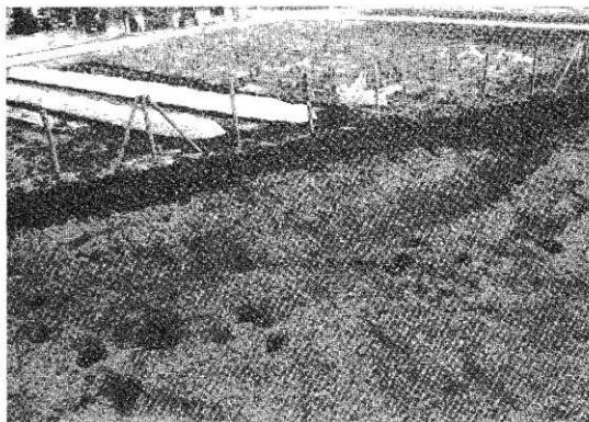
第6号古墳跡
