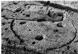
第91号住居跡
