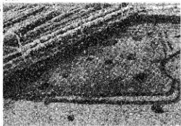
第28号住居跡
