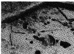
第6号住居跡
