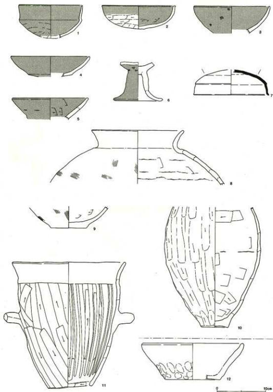
第401図 第52号住居跡出土遺物
