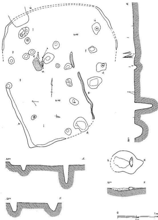
第369图 第42·43号住居跡
