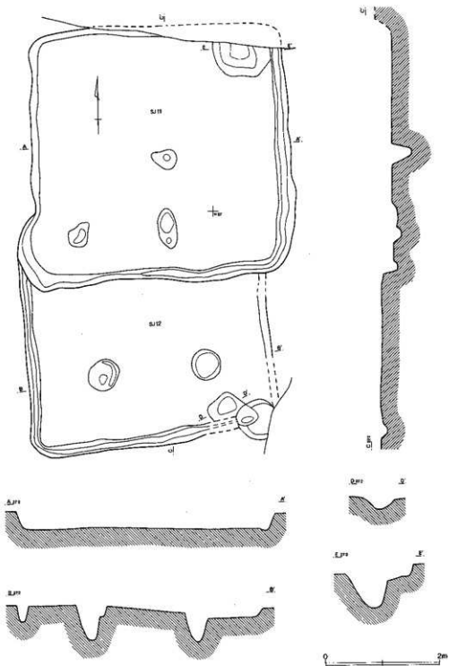
第359圖 第11・12号住居跡
