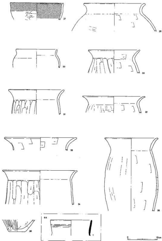
第354图 第5号住居跡2、第6号住居跡出土遺物
