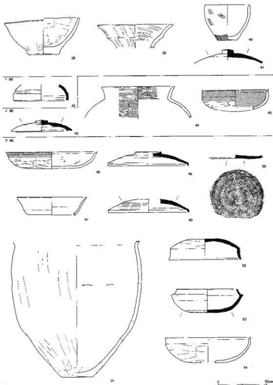
第485図 グリッド出土遺物③
