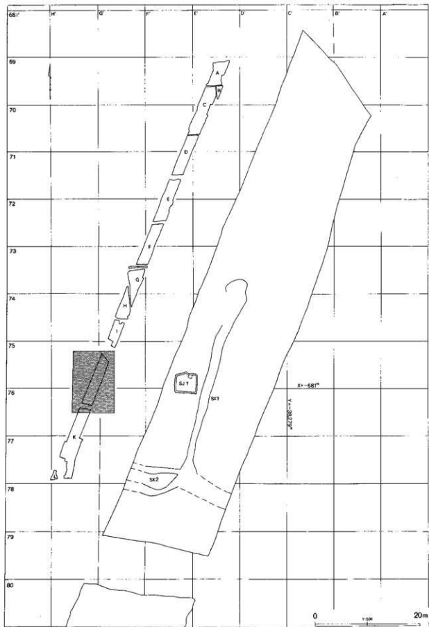
第337圖 全測図田
