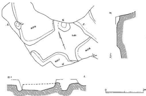
第413図 第61号住居跡
