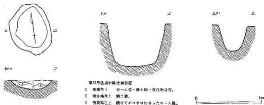
第403図 第53・54号住居跡②
