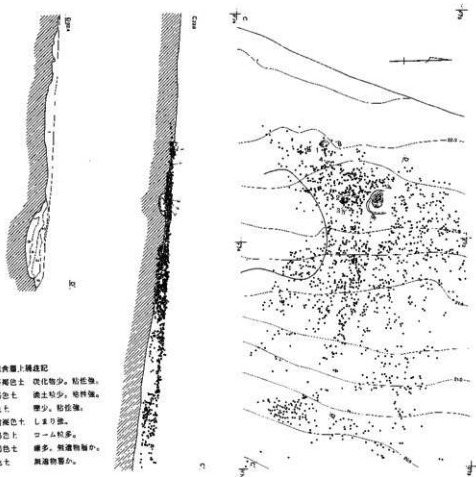
第445図 J区包倉層
