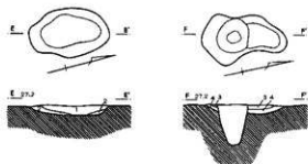
第379図 第31、33 35号住居跡②
