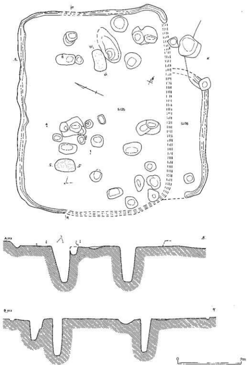
第427图 第25·26号住居跡(1)
