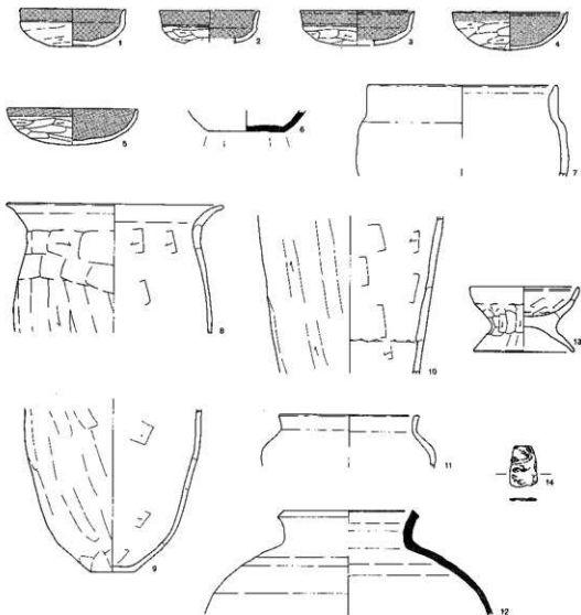
第368図 第17号住居跡出土遺物
