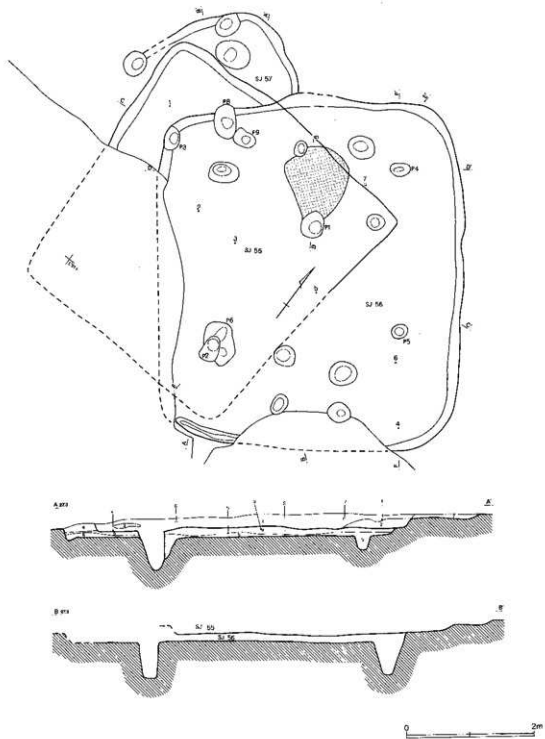
第408图 第55~57号住居跡(1)
