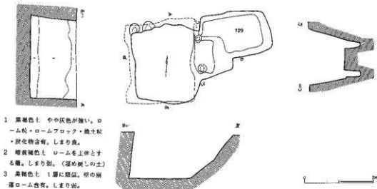
第444図 地下式坑
