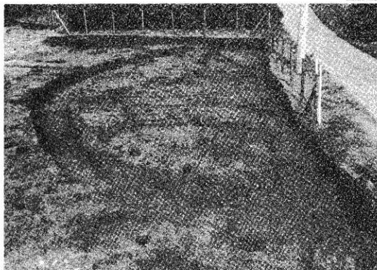
第4号古墳跡
