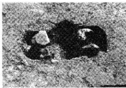
第1号火葬墓
