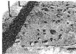
第85号住居跡
