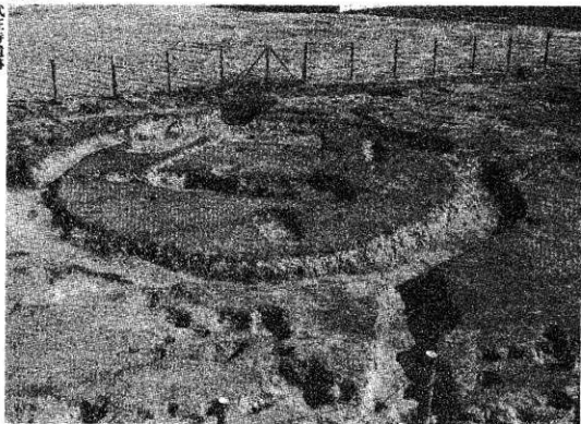
第10号古墳跡
