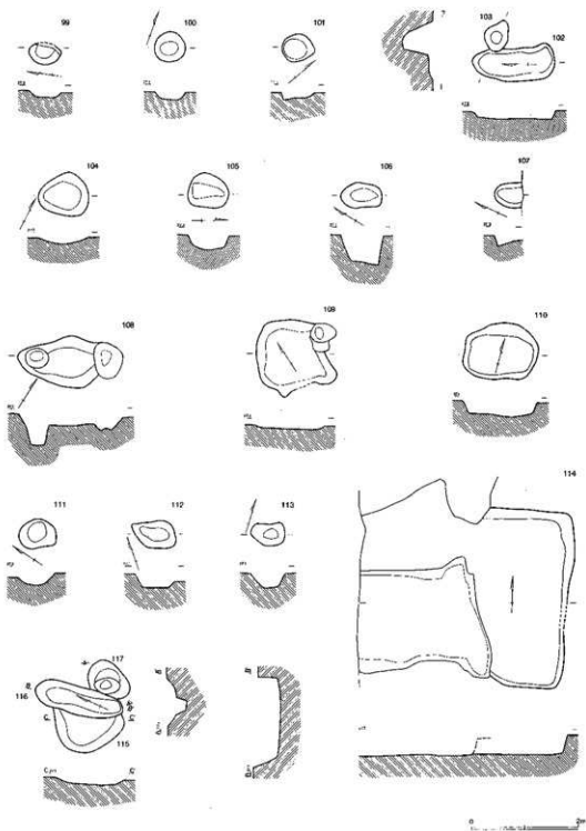
第452图 土壤B
