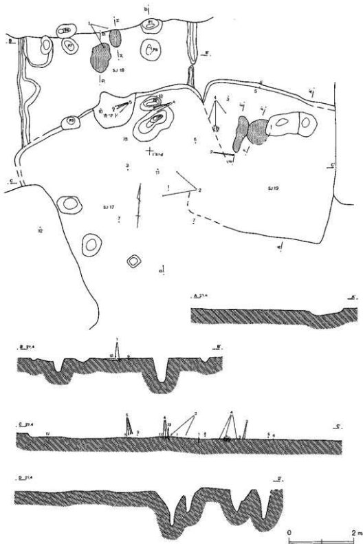
第364图 第17~19号住居跡(1)
