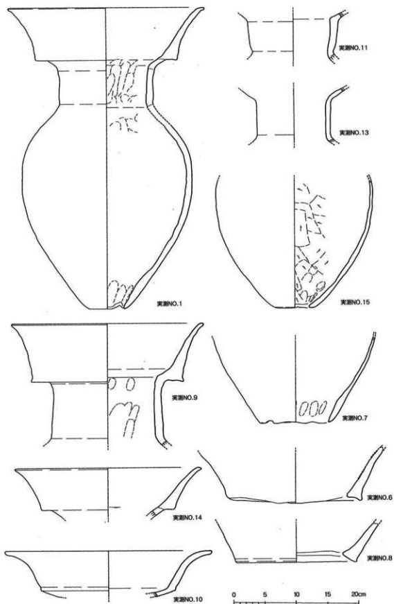
第10図 遺物実測図 1
