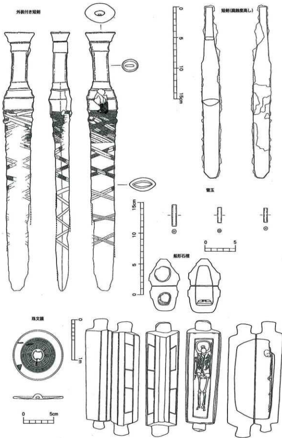
第12図 経塚古墳出土遺物実測図
