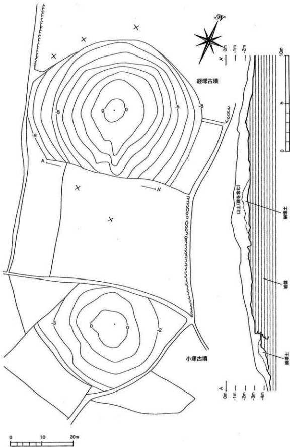
第3図 墳丘測量図(昭和26年)
