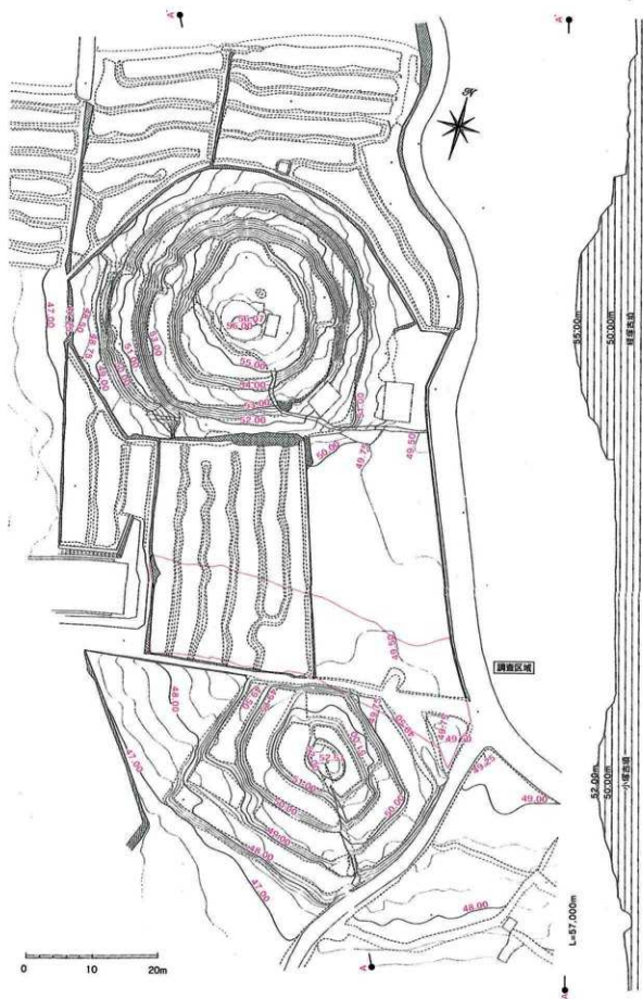
第2図 墳丘測量図(平成9年)
