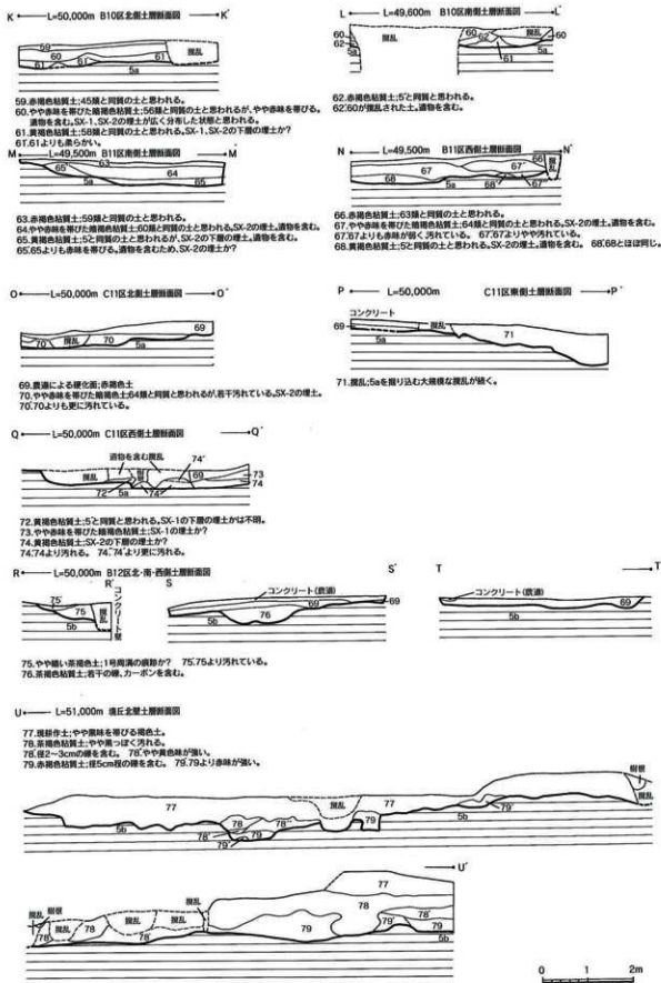
第7図 土層断面図 3
