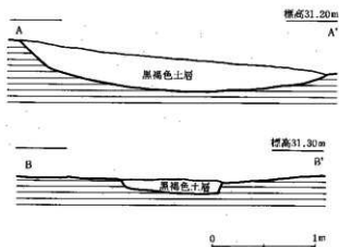
Fig. 11 周溝断面実測図 (1/40)
