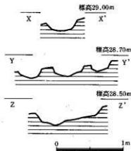
土坑 1は1号墳南西側で周溝に接して検出された。 Fig. 14 溝断面実測図(1/40)
