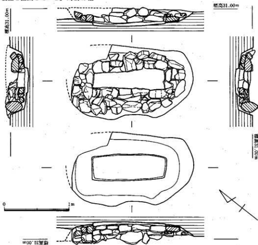
Fig. 12 2号墳主体部実測図 (1/30)
