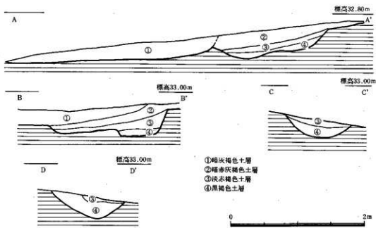
Fig. 5 周溝断面実測図 (1/40)
