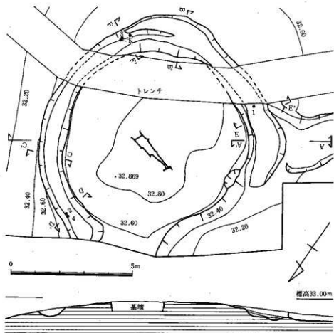
Fig. 4 1号墳墳丘測量図 (1/100)
