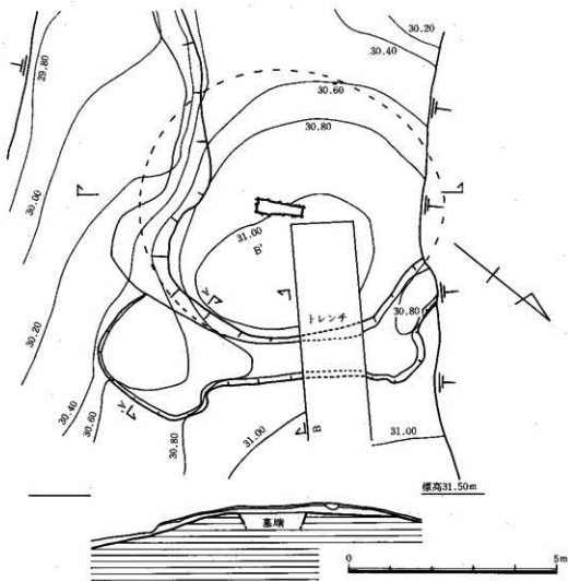
Fig. 10 2号墳丘陵測量図 (1/100)
