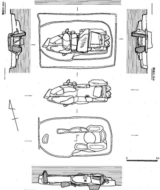
Fig. 7 1号墳主体部実測図(1/30)
