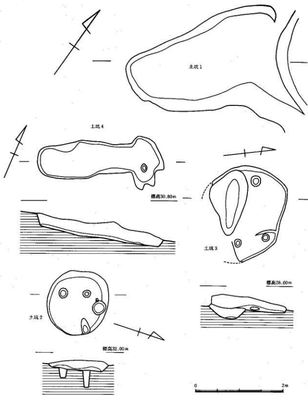
Fig. 15 土坑実測図 (1/40)
