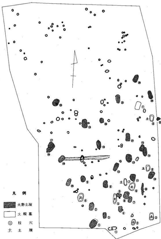
第3图 上町木下遺跡調査区内遺構配置図 (1 / 150)
