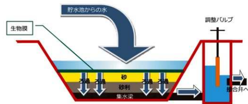
緩速ろ過の仕組み
