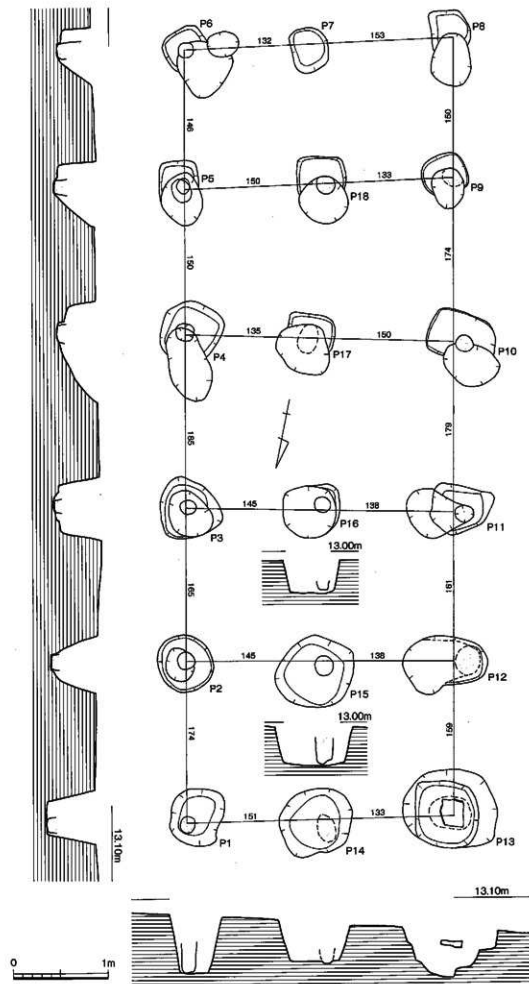
第13図 C-6-谷地点1号建物実測図 (1/60)
