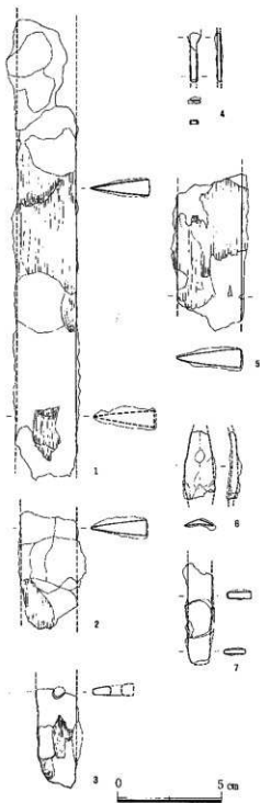
第6図 六部山5号墳出土遺物実測図(1)
