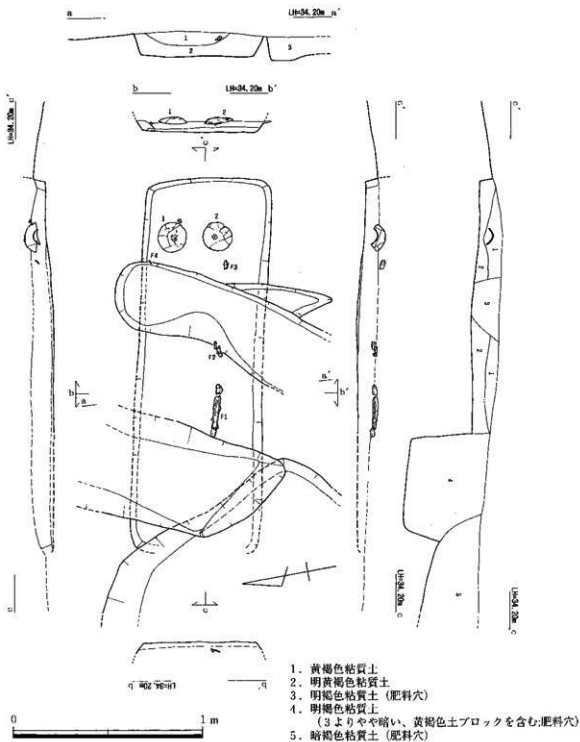
第5図 六部山5号墳埋葬施設実測図
