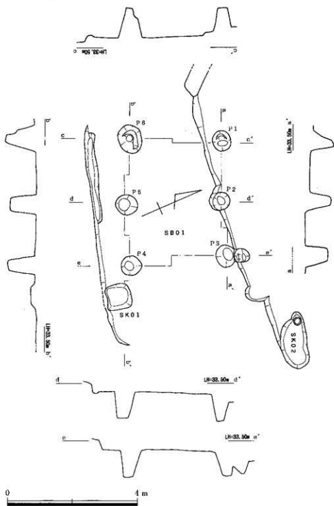
第14图 SB01平面图
