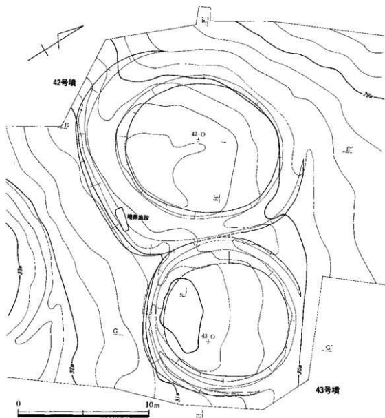
第10図 六部山42・43号墳墳丘実測図
