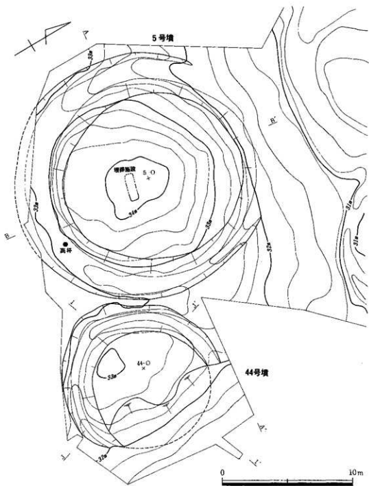
第4圖 六部山5・44号墳 墳丘実測図
