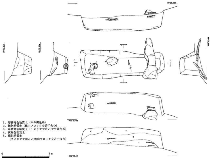
第12図 六部山42号墳周溝内埋葬施設実測図
