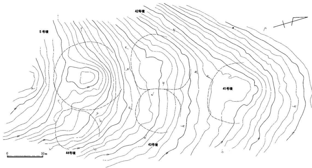
第17图 六部山41・42・43・44・5号墳地形実測図
