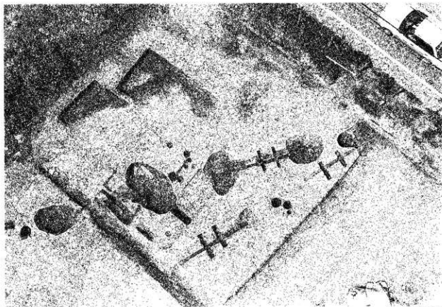
2 製鉄炉全景
