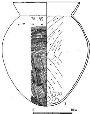
第8図 SD02出土土器実測図 (1/4)
