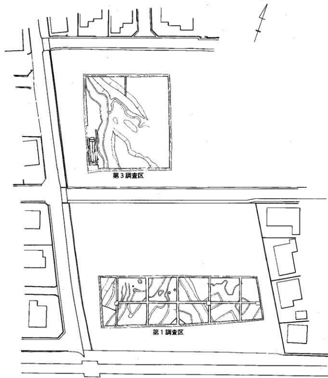
第4図 西・老丁田遺跡遺構位置図 (1/600)
