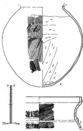
第13図 SD06出土土器実測図(6:1/2 7:1/2)
