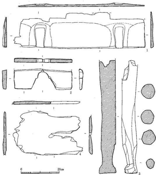
第10图 第1区出土木制品实测图 (1/6)
