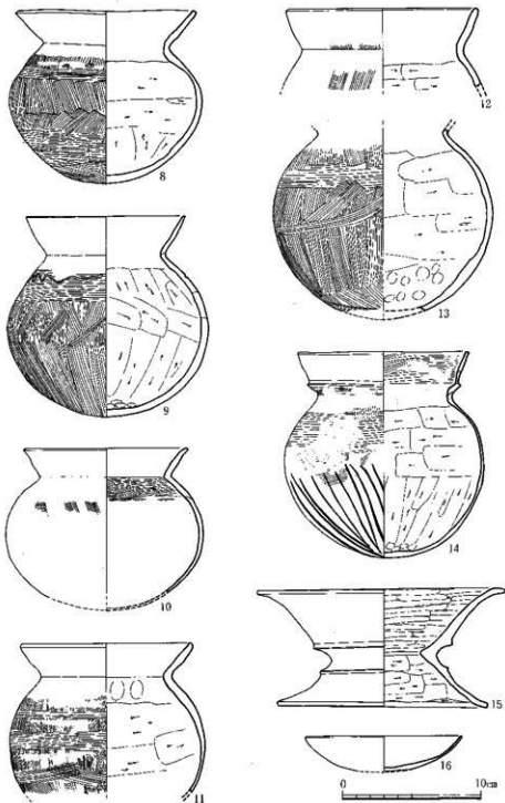
第14图 SD08出土土器实测图 (1/5)
