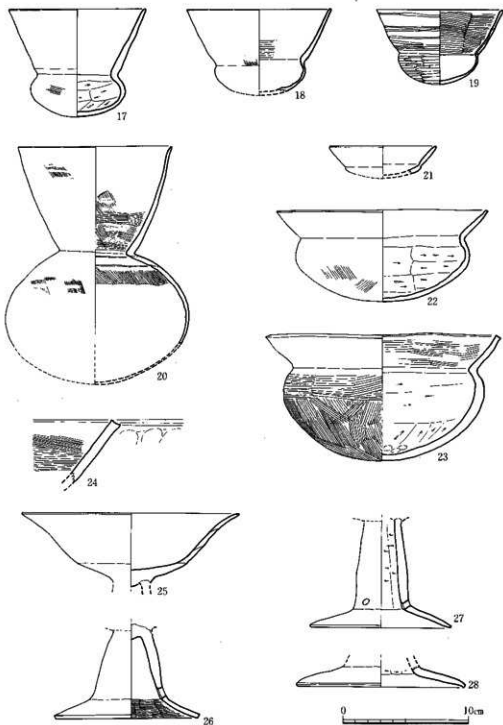
第15图 SD08出土土器实测图(1/4)
