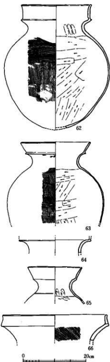
第25図 SD08出土土器実測図 (1/6)
