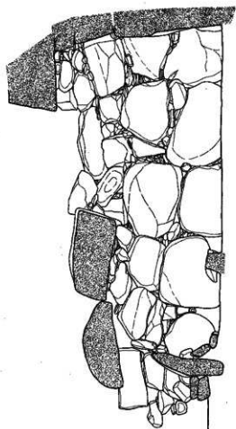
尾花屋敷2号墳石室実測図 (1/50)
