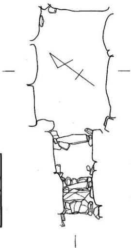
尾花屋敷2号墳石室実測図 (1/50)
