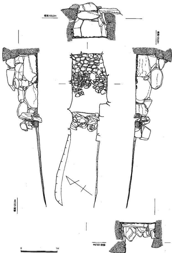
尾花屋敷6号墳石室実測図 (1/30)
