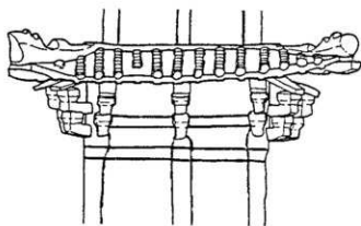
I類 (例) 萬蒲沢遺跡 (1/6, 鳥羽ほか 1997—部修正)
