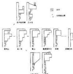
模式図による斗栱の変化 (高崎 1989)
