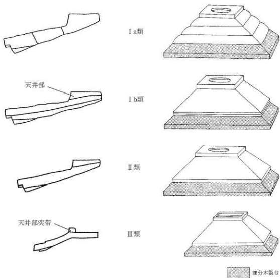
第1図 屋蓋部製作技法（関東地方）
