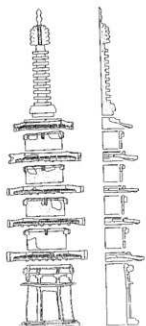
(例) 谷津遺跡 (1/16. 田中 池田ほか 2000一部加筆)
