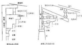
瓦塔の斗栱表現模式図 (松本 1983)
