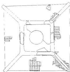
(例) 大仏廃寺③ (1/6. 宮道 1992)
