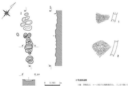
第6図 2号道路遺構 (1/60)、出土遺物 (1/3)
