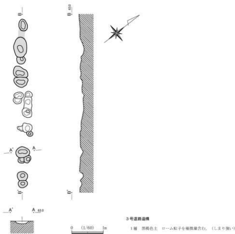
第7図 3号道路遺構 (1/60)
