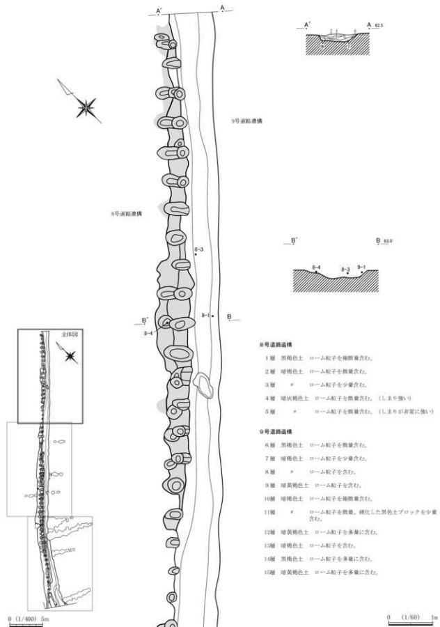
第12図 8、9号道路遺構 (1) (1/60)
