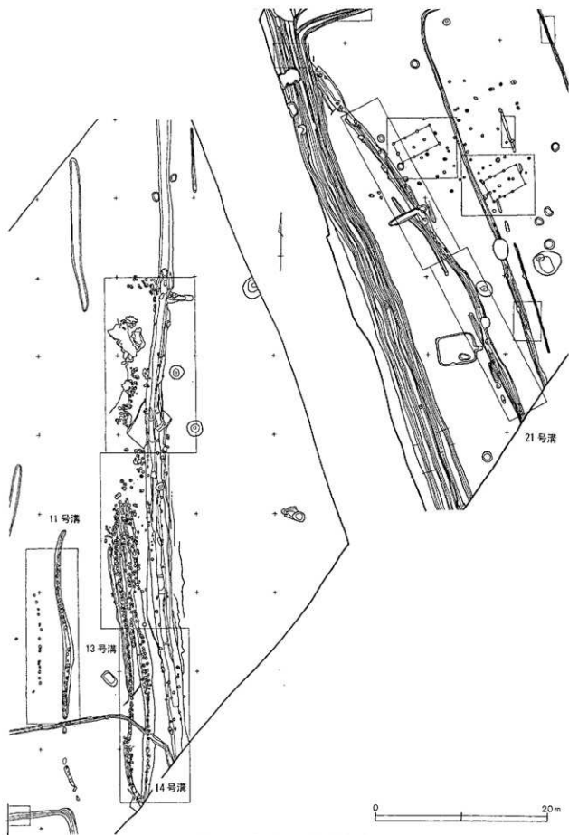
第17图 下向山道跡道路遺構 (1/400)
