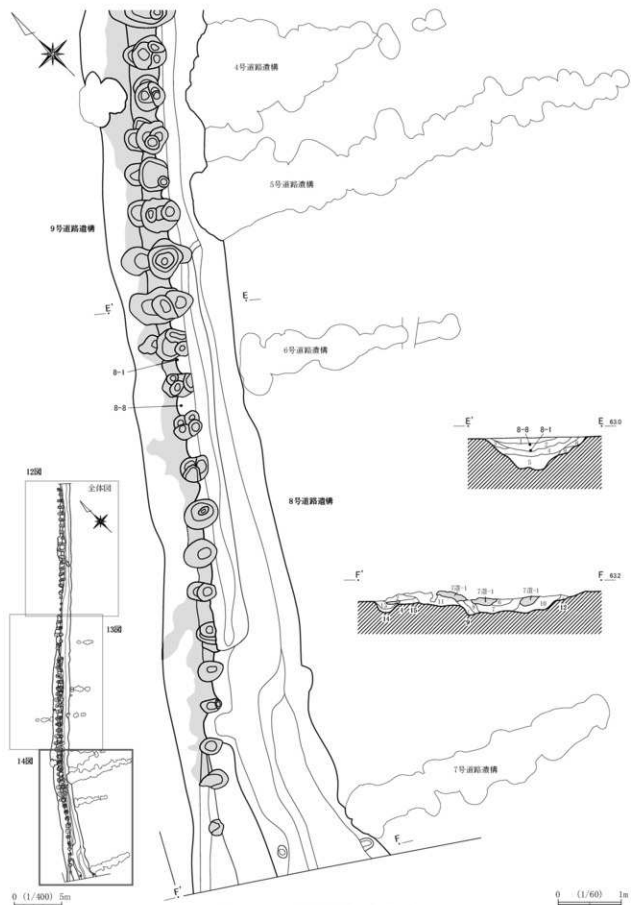
第14图 8、9号道路遺構(3) (1/60)
