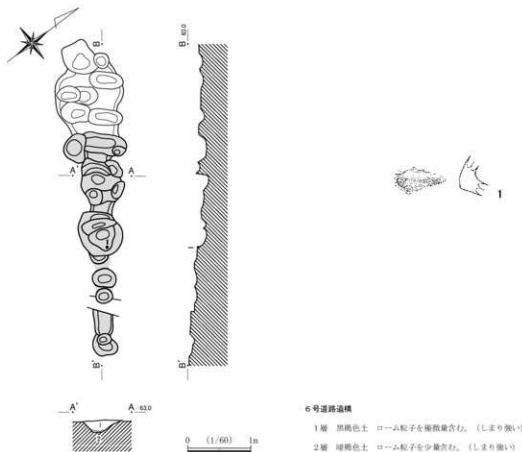
第10図 6号道路遺構 (1/60)、出土遺物 (1/3)
