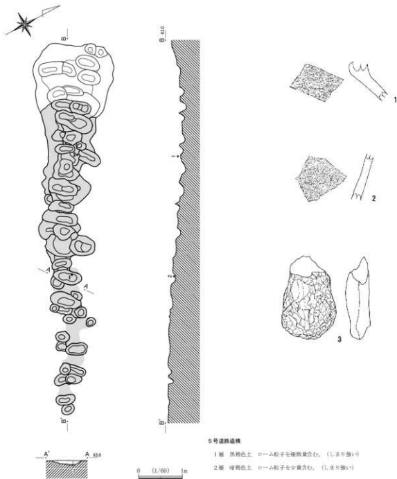
第9図 5号道路遺構 (1/60)、出土遺物 (1/3)
