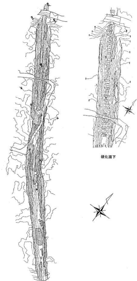
第16図 向谷遺跡道路遺構 (1/600)、硬化面下は (1/200)
