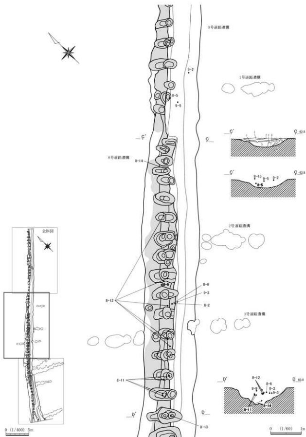
第13图 8、9号道路遺構(2) (1/60)
