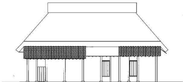
北側立面图 (1:150)
