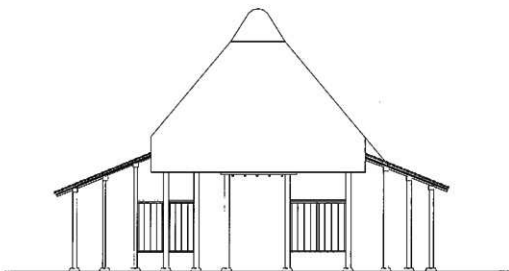
西侧立面图 (1:150)
