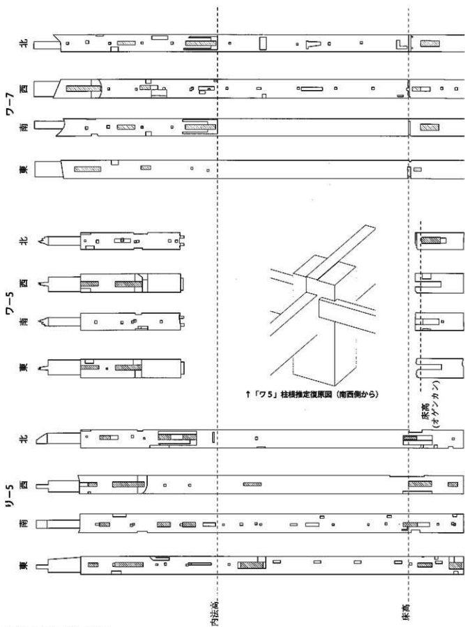
↑柱4面横断図 松材 その2
