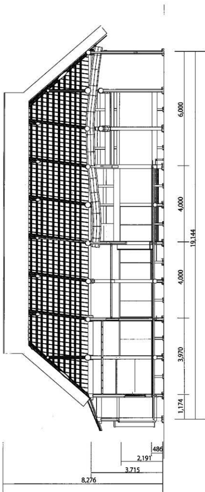
縦断面図 (1:100)
