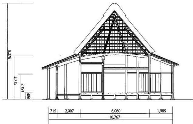
土間横断面図 (1:100)
