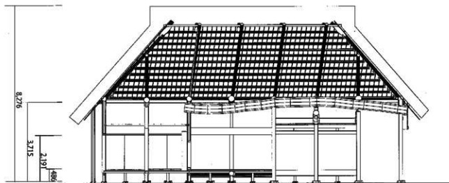
縦断面図 (1:125)
