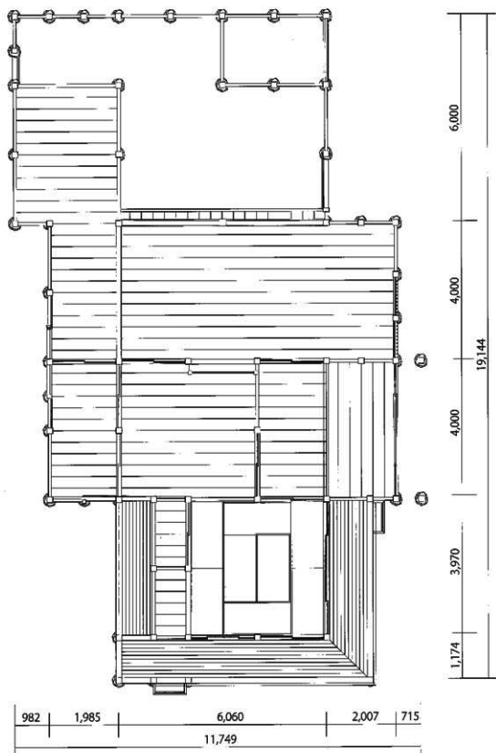
平面図 (1:100)
