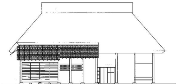
南侧立面图 (1:150)
