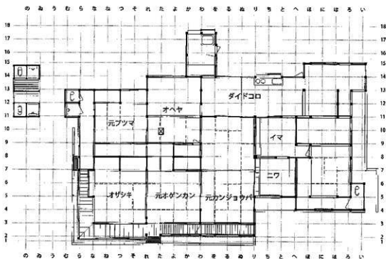
↑解体前平面図
