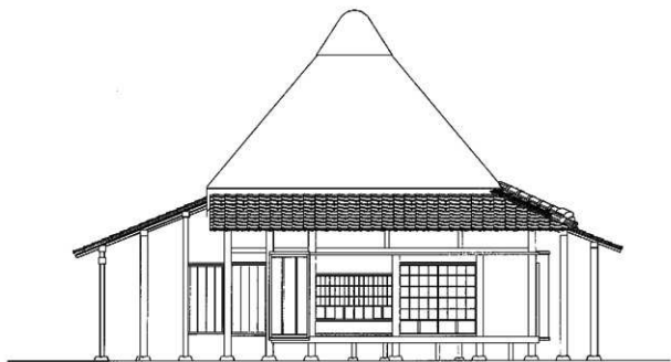
東側立面圖 (1:100)
