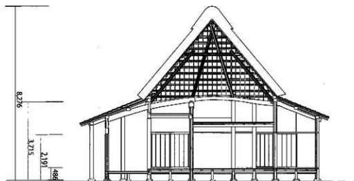
土間横断面図 (1:125)
