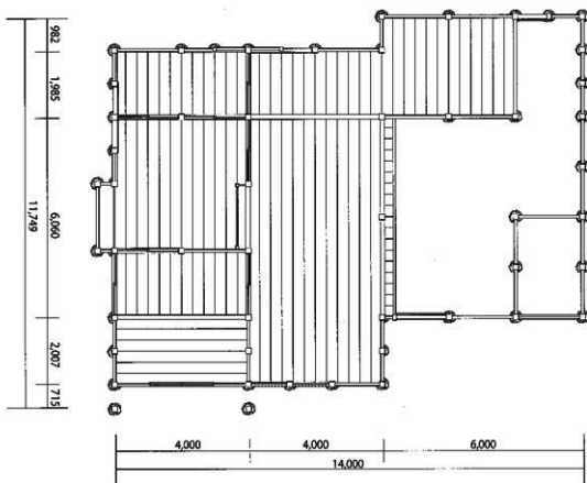
平面図 (1:125)
