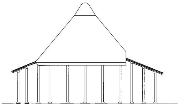
西側立面圖 (1:100)
