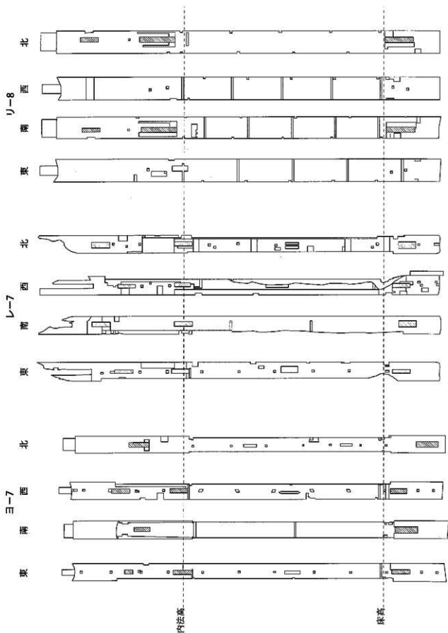
↑柱4面透視図 松材 その3
