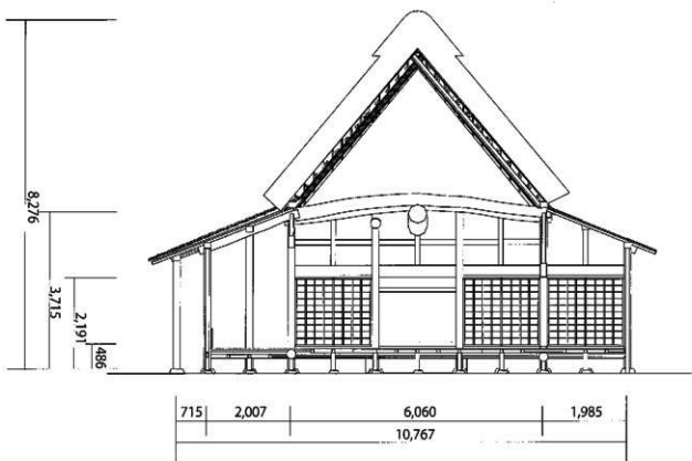
玄関横断面図 (1:100)
