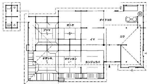
↑大正初期推定復原平面図
