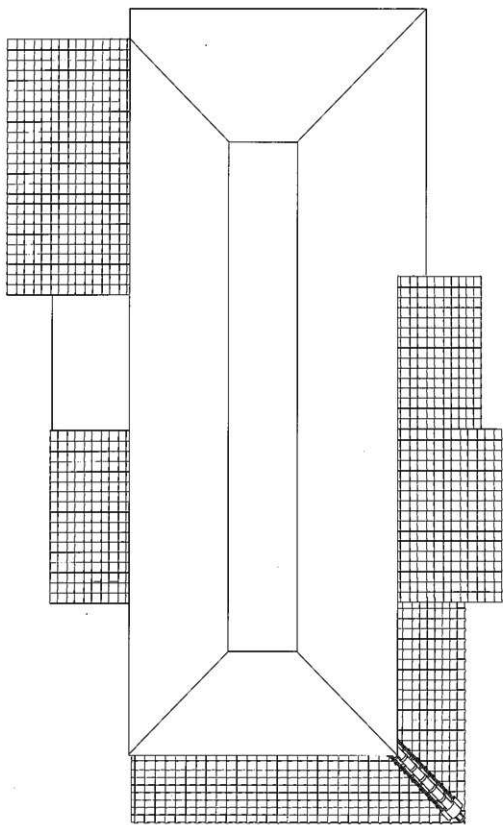
屋根伏图 (1:100)
