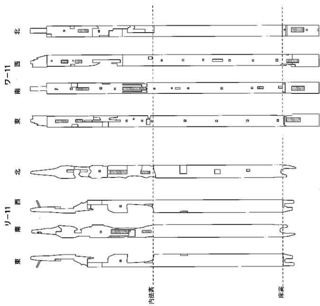
↑柱4面透視図 松材 その5
