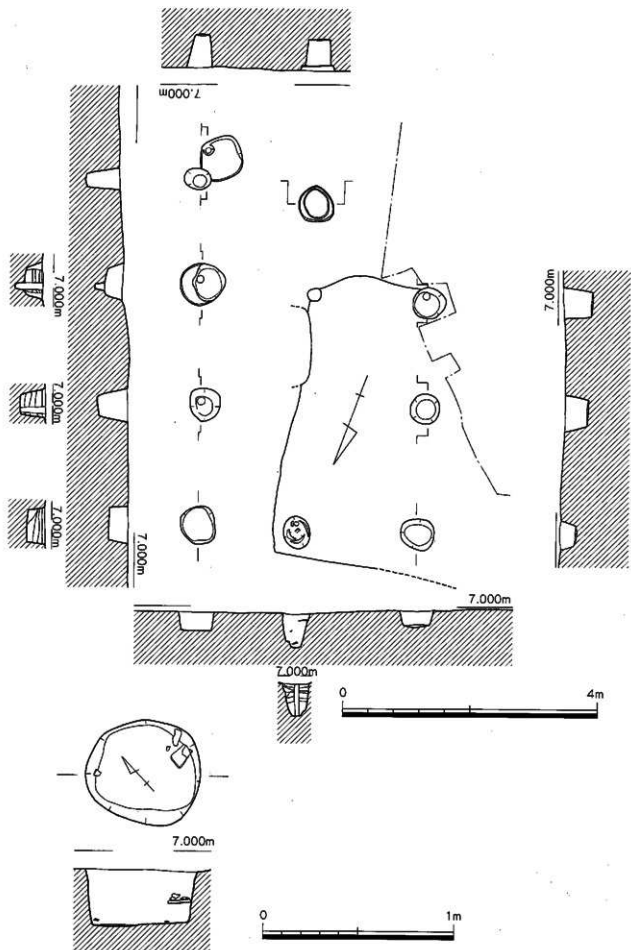
第7图 A区1号掘立柱建物平面美测图 (1/60·1/20)
