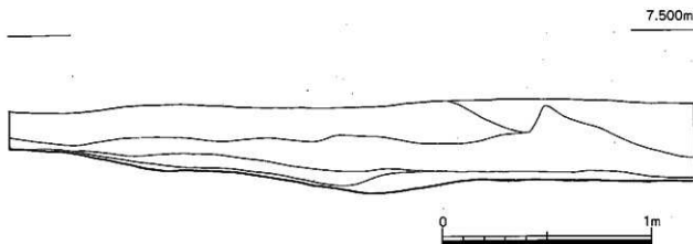
第3図 前原西町遺跡2 A区基本層序土層断面実測図 (1/20)
