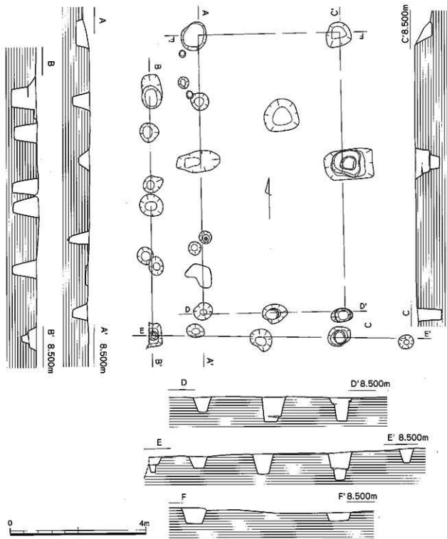
第14图 B区 近世掘立柱建物实测图 (1/80)
