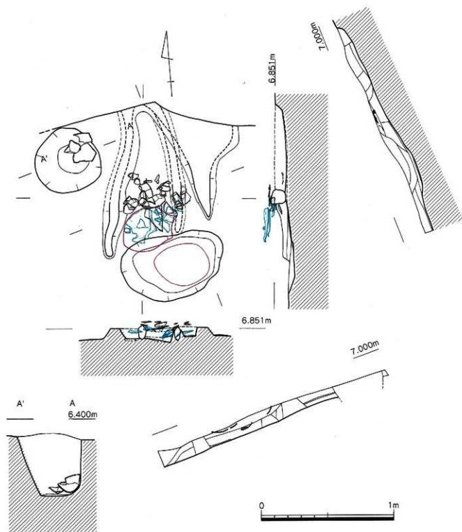
第6図 A区1号竪穴式住居カマド平断面実測図 (1/20)
