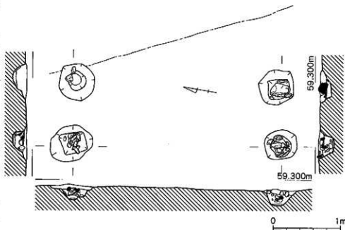
第14図 1号堀立柱建物実測図(1/40)
