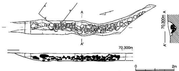
第22図 6号溝実測図 (1/60)
