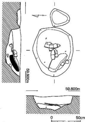
第18図 焼土坑実測図(1/20)
