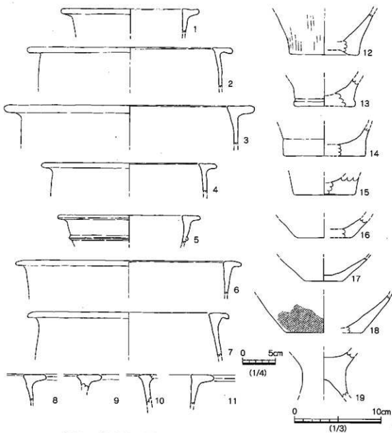
第26図 未永数蔵町・梅木田遺跡出土弥生土器実測図(1/3、1~7は1/4)
