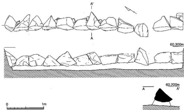
第17図 石垣状遺構断面実測図 (1/30)
