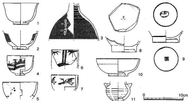
第10図 1号井戸出土遺物実測図(1/3)
