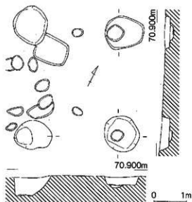
第23図 1号堀立柱建物実測図 (1/40)
