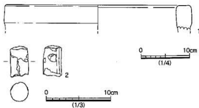
第6図 1号埋桶出土遺物実測図(1/3、1/4)
