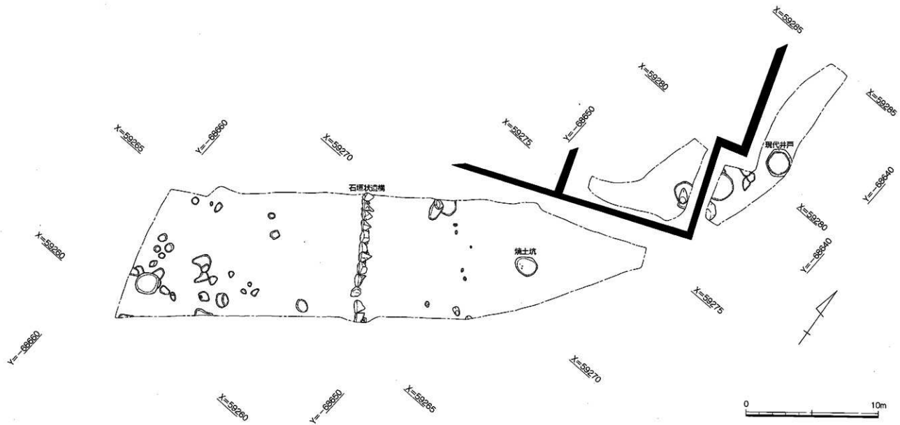
付図2 米承敷藤町遺跡 D地区 全体図(1/100)
