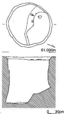
第9図 1号井戸実測図(1/30)
