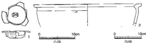
第25図 208・168号ビット出土遺物実測図(1/3, 2は1/4)
