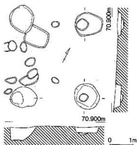
第23図 1号堀立柱建物実測図 (1/40)
