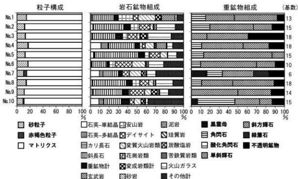
第2図 土器胎土の岩石鉱物組成
