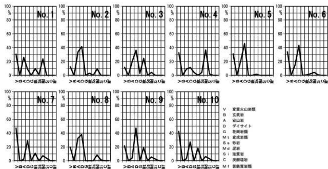
第3図 岩石組成折れ線グラフ
