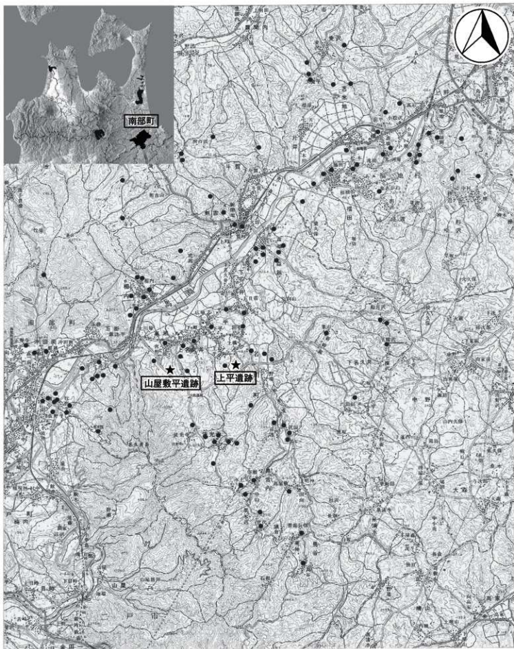
図1 遺跡位置
