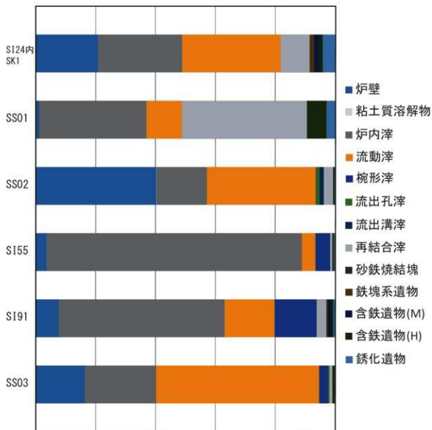
図175 製鍊炉・排滓場出土遺物重量割合
