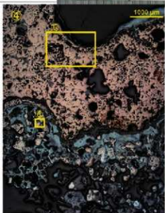
写真2 炉内滓の顕微鏡組織
