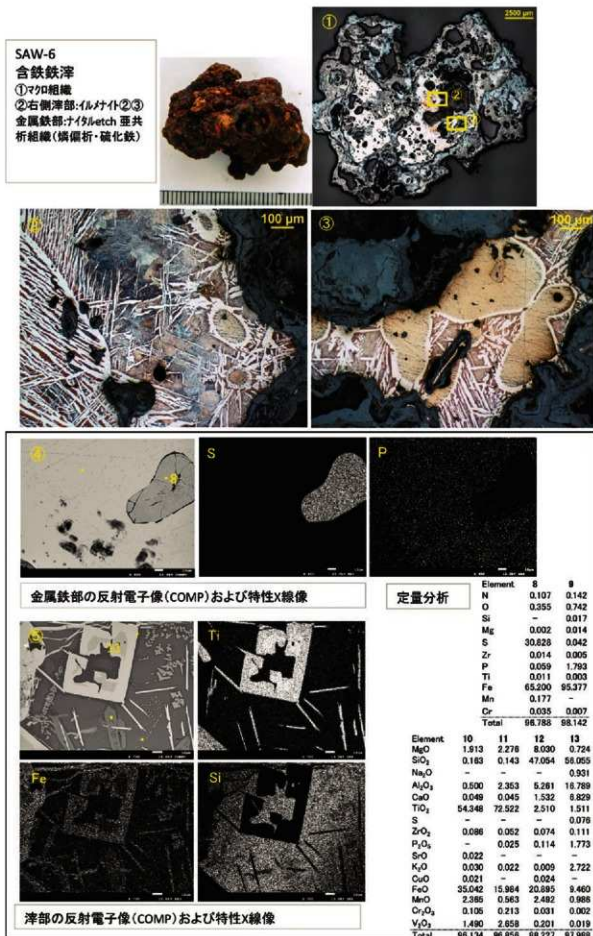
写真4 含鉄鉄滓の顕微鏡組織・EPMA 調査結果
