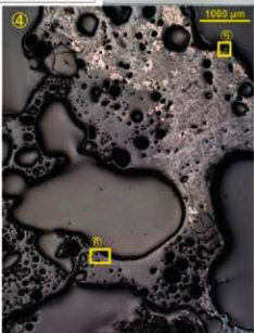
写真1 流動滓・炉内滓の顕微鏡組織
