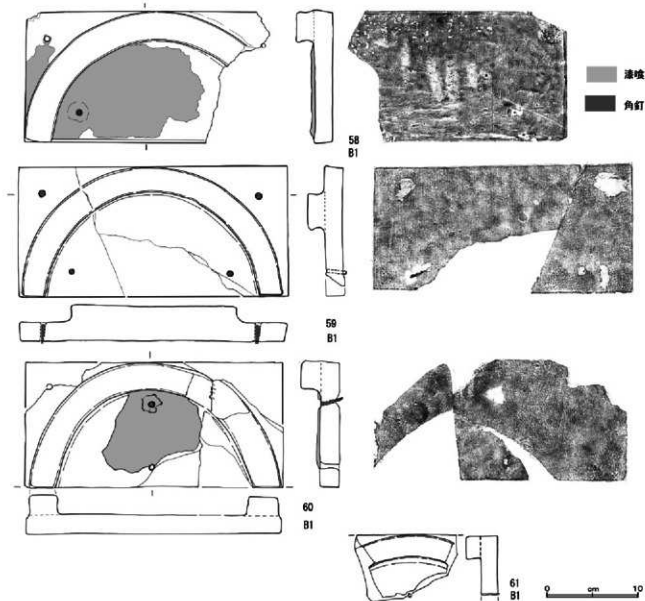
第15図 瓦(7) 棟飾瓦
