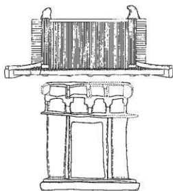
第2図 瓦堂 (1. 埼玉県若宮遺跡出土 2. 千葉谷津遺跡出土)
