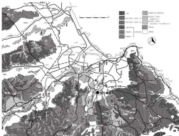
図4 八戸市付近の段丘区分図（松山 1983 を再トレース）
