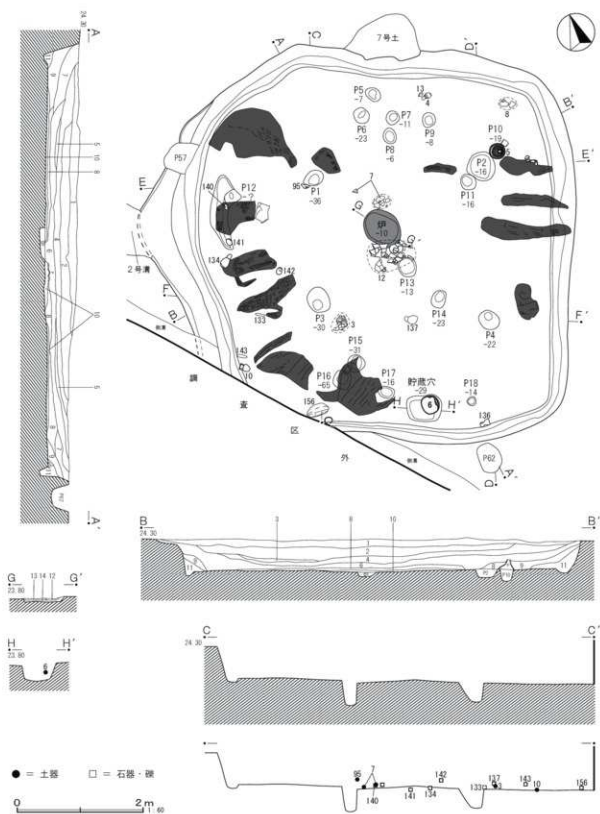
第17図 第3号住居跡(1)
