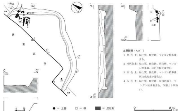
第49図 第8号住居跡
