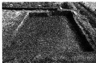
NR27 (56T 部分) As-B 下面検出状況 西から
