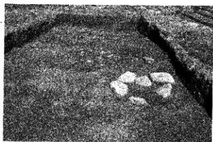
SB01 A1 礎石据付穴・SX06 検出状況 南から
