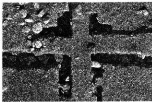
SB03 C8 柱筋交点 オルソソ画像 上が北
