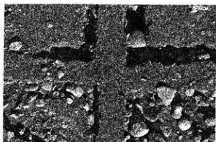
SB03 D8 柱筋交点 オルソソ画像 上が北
