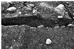
SB03 北辺 (49-49' 北寄り) 基壇断面 東から
