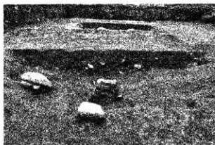
SD23 (60T B-B') 断面 西から
