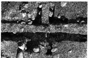
SB03 B5 柱筋交点 オルソソ画像 上が北
