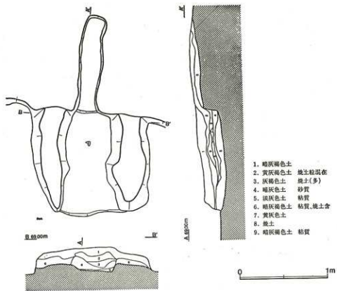
第200図 4号住居跡カマド
