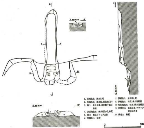
第213図 10号住居跡カマド
