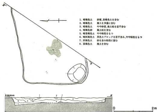
第233図 23号住居跡
