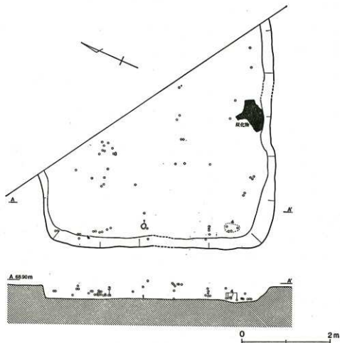
第216図 11号住居跡
