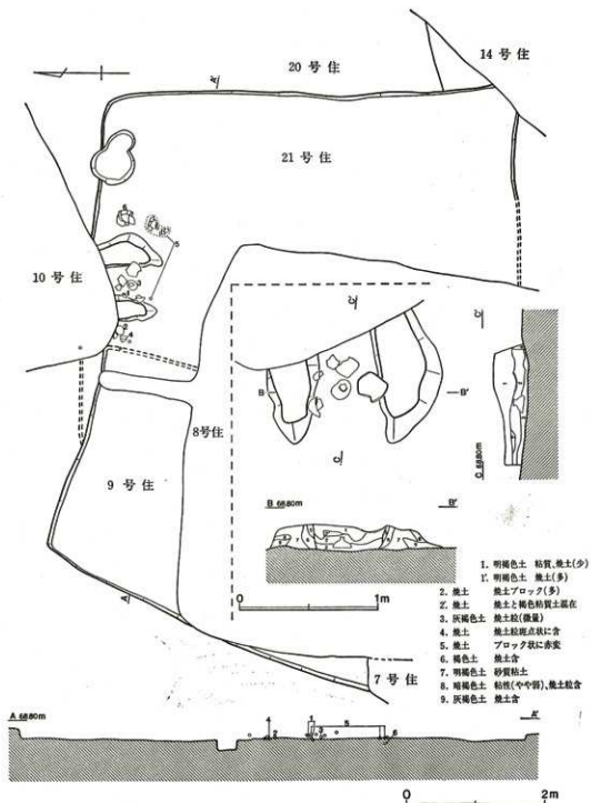
第211図 9・21号住居跡、21号住居跡カメラ
