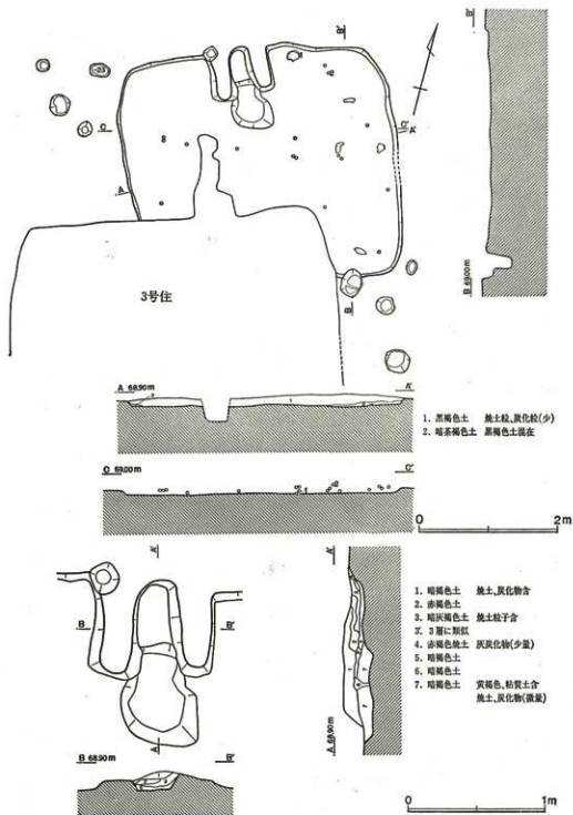
第193図 2号住居跡・カマド
