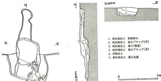
第196図 3号住居跡カマド
