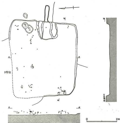
第199図 4号住居跡
