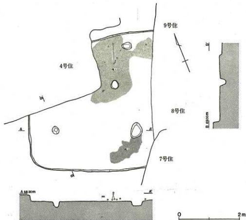
第203図 5号住居跡
