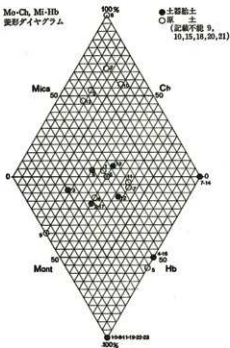
Mo-Mi-Hb 三角ダイアグラム
