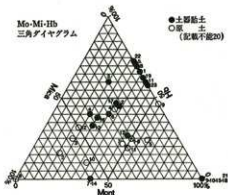
Fe-Mn-Ti 三角ダイアグラム
