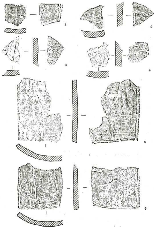
第270图 瓦尖剖面图
