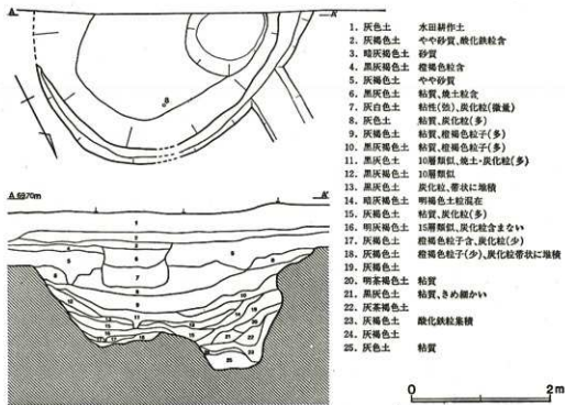
第244図 1号井戸跡
