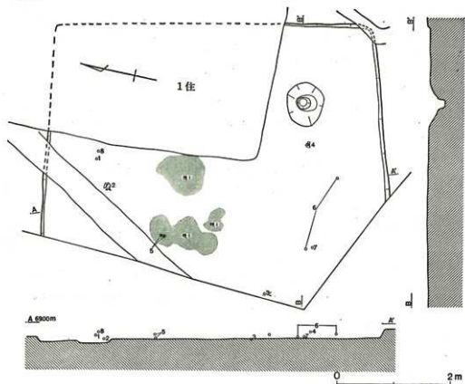
第241図 30号住居跡
