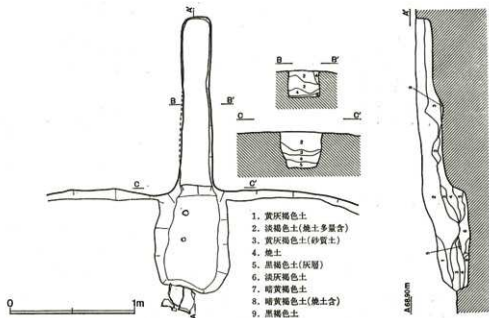
第209図 8号住居跡カマド
