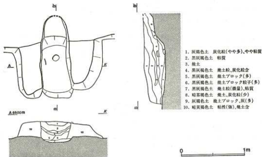
第223図 14号住居跡カマド
