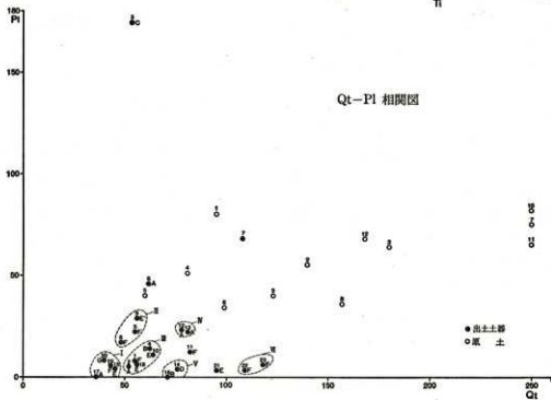
第272図 三角・菱形ダイアグラム、Qt—Pi 相関図
