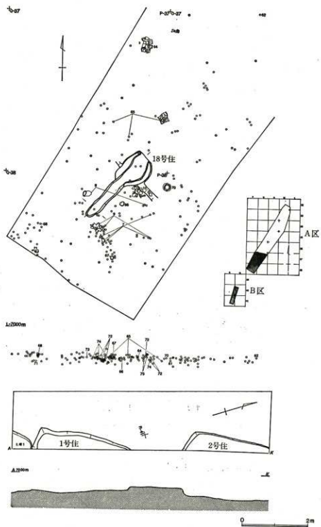
第259图 B区遗物分布图(3)、A区1・2号住居跡
