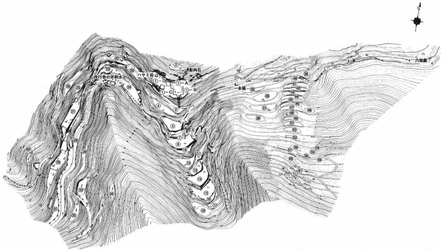
第3図 松尾寺遺跡坊跡調査 平面図 S=1:2,000
