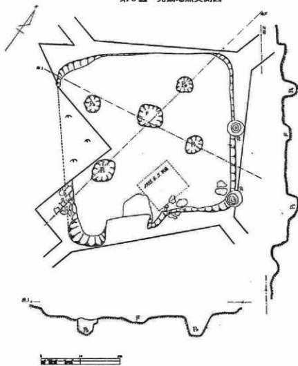
第4图 竖穴住居跡实测图
