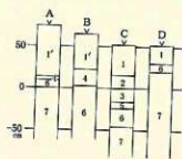
土層柱状図
