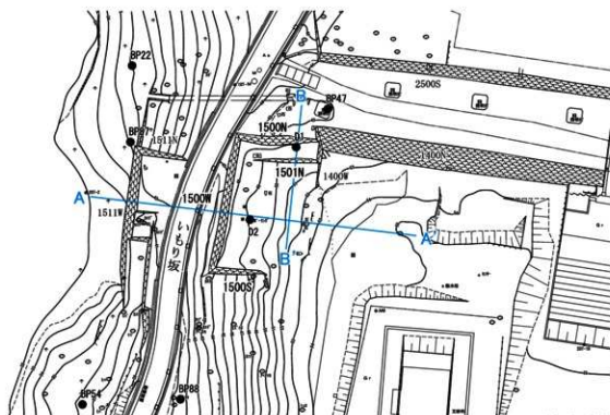
現況平面図
