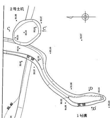
2号土坑・1号溝平面図(S=1/40)
