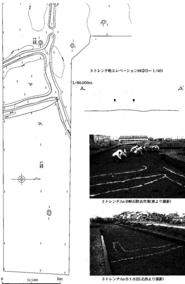
第8図 3 トレンチ平面図②(S=1/100) 畦エレベーション図②(S=1/40)
