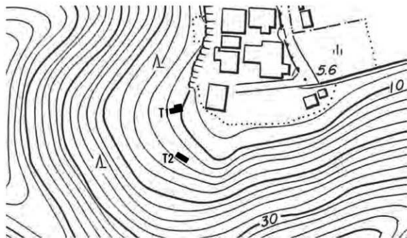
第13図 八戸地区トレンチ位置図 (S=1/1,000)
