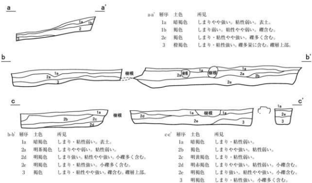
第20図 三上寺跡トレンチ土層図 (S=1/80)
