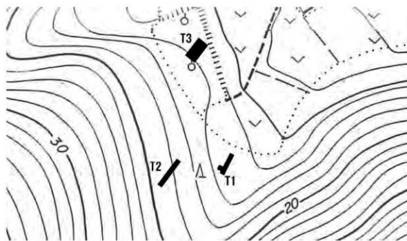
第4図 迫田地区トレンチ位置図 (S=1/1,000)
