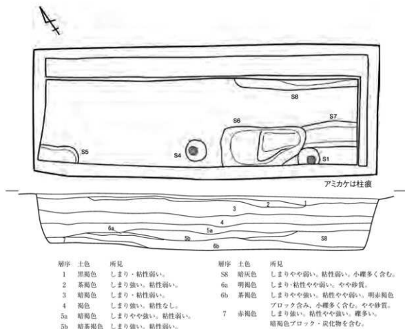
第15図 八戸地区T2平面図・北東壁土層図 (S=1/40)
