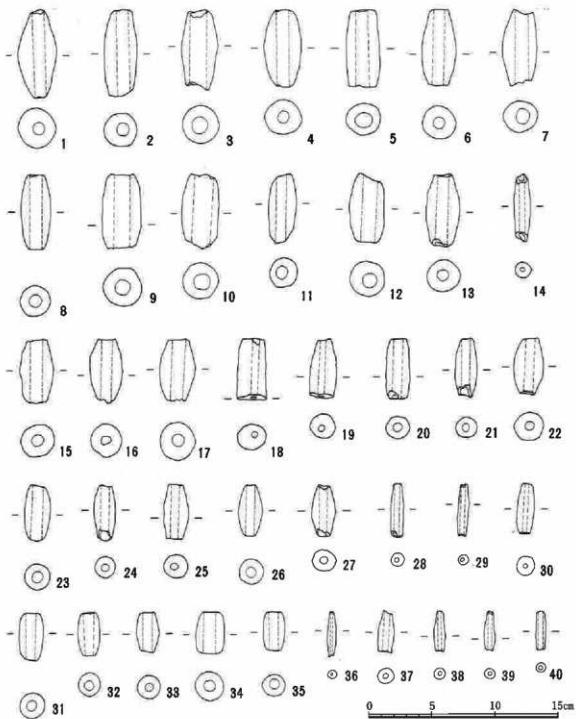
第13图 出土遺物(土錘)实测图
