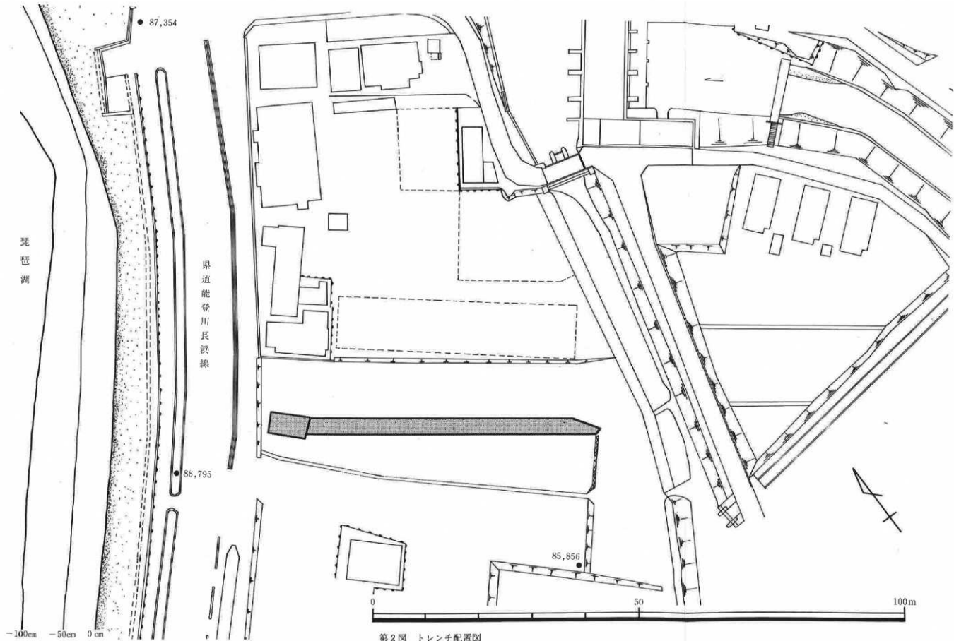
第2図 トレンチ配置図
