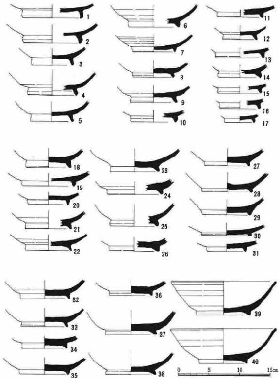
第10图 出土遗物(土器)实测图(4)
