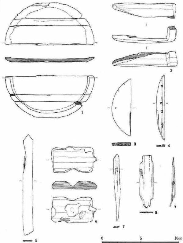
第15図 出土遺物(木器)実測図
