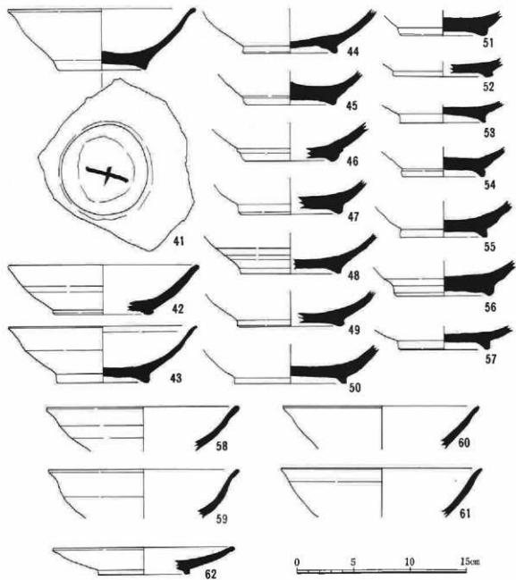
第11图 出土遗物(上器)实测图(5)
