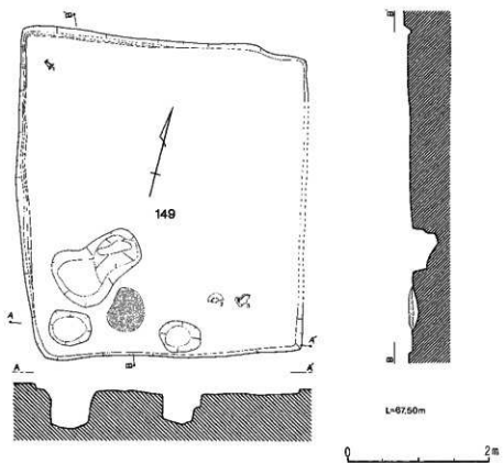
第299図 149号住居跡
