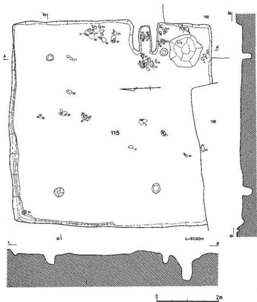
第256图 115号住居跡
