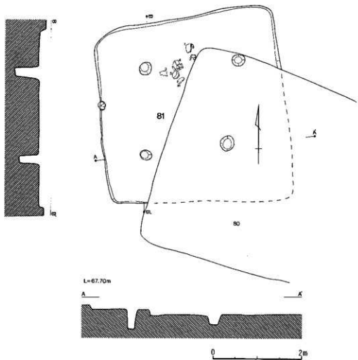
第183图 81号住居跡
