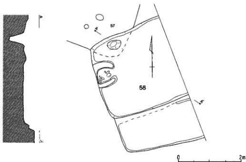
第145图 58号住居跡
