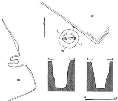
第332图 1号井戸跡
