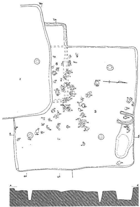
第7图 3号住居跡
