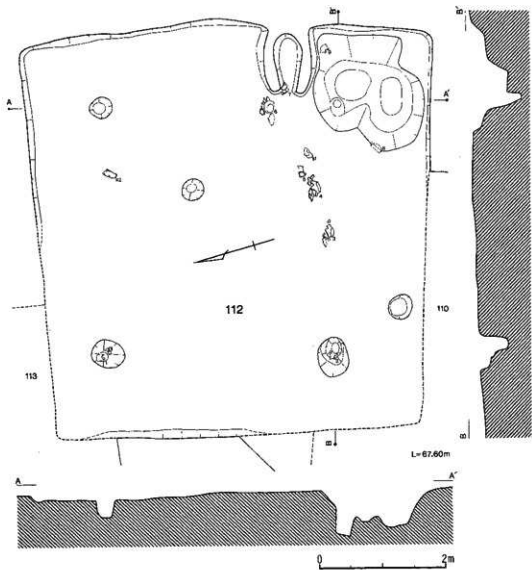
第253图 112号住居跡
