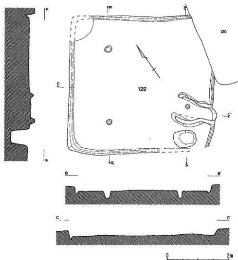
第269图 122号住居跡
