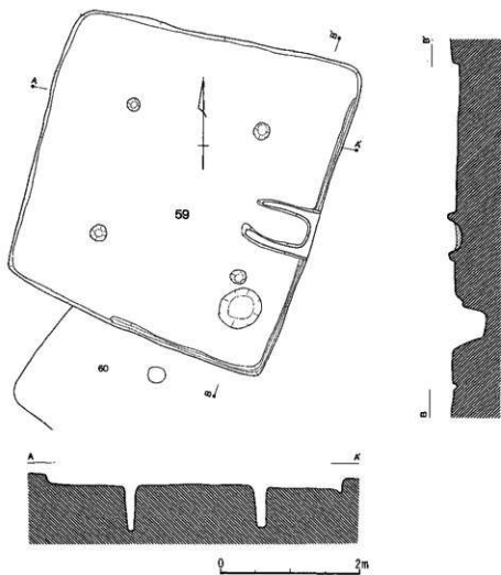
第148图 59号住居跡
