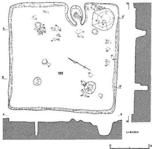
第304图 151号住居跡
