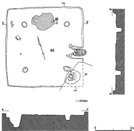
第186区 83号住居跡
