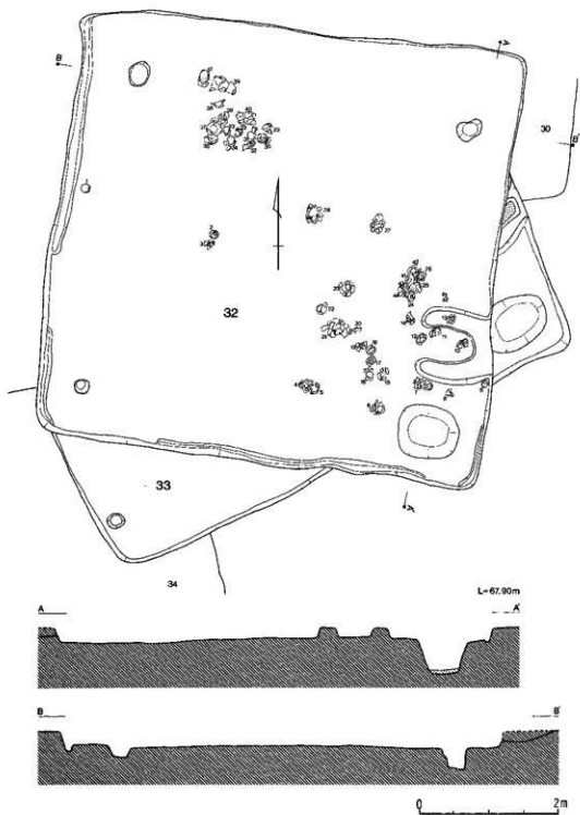
第86図 32号・33号住居跡
