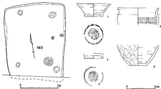
第315图 163号住居跡
