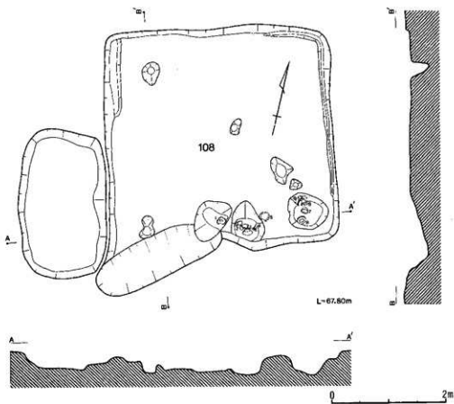
第245图 108号住居跡
