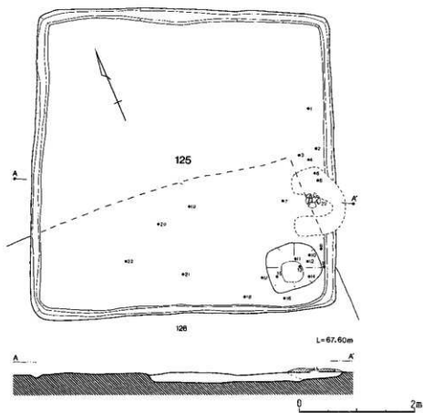
第277图 125号住居跡
