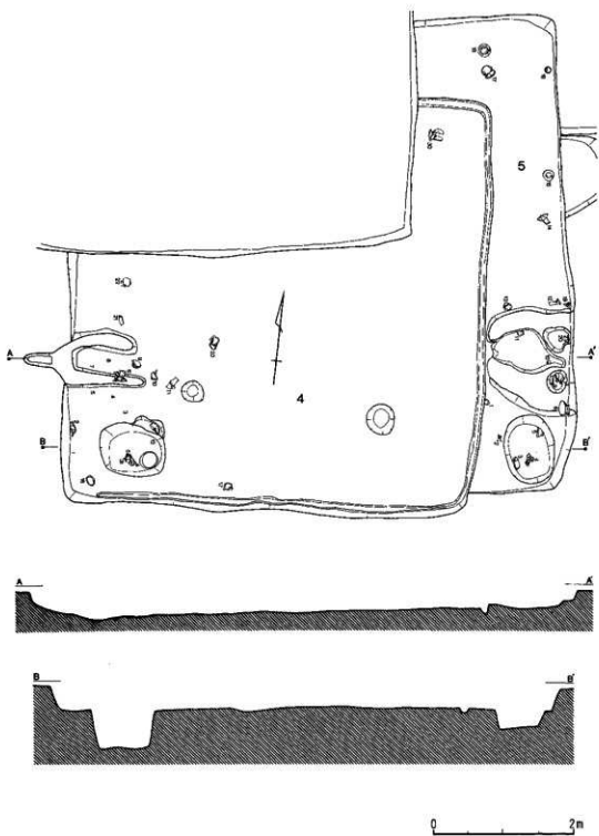
第14图 4号·5号住居跡
