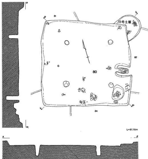
第180图 80号住居跡
