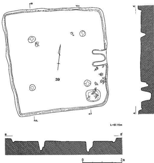
第102图 39号住居跡
