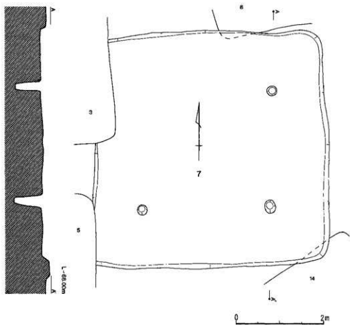
第21图 7号住居跡
