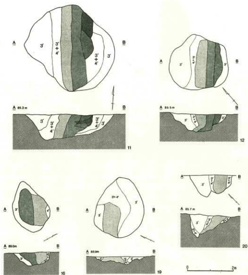
第104図 鶴巻遺跡風倒木痕1類
