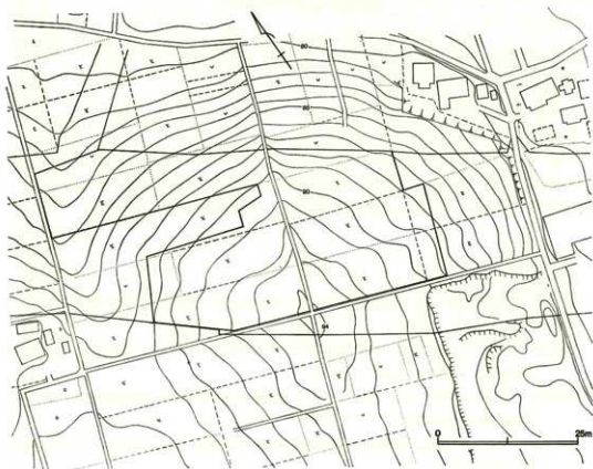
第87図 中井丘遺跡全測図
