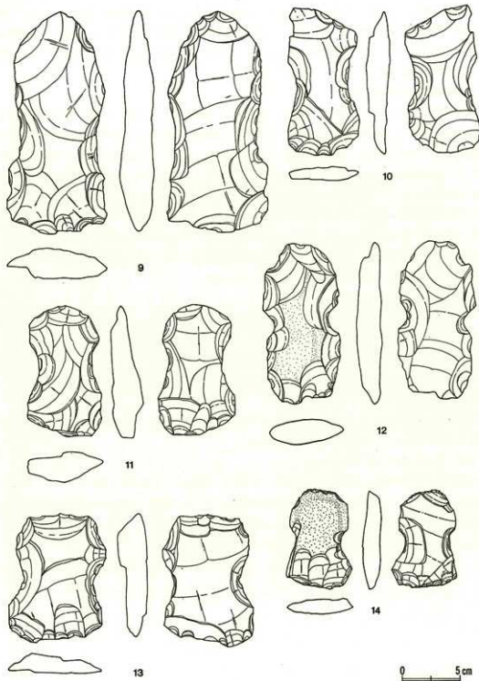
第112図 グリッド出土石器実測図(3)
