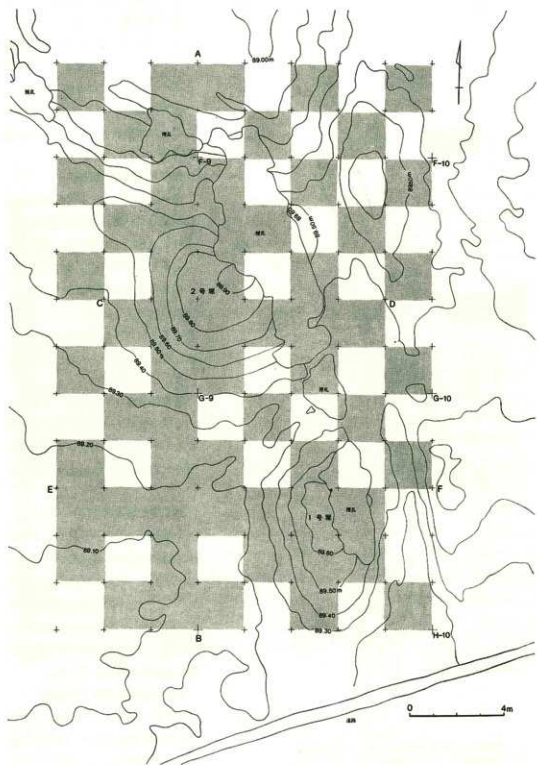
第101図 鶴巻遺跡1・2号窟全測図
