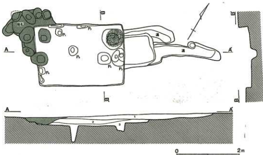
第6図 第1号住居址実測図
