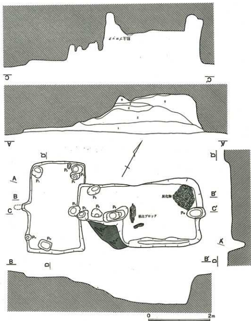
第8図 第2号住居址実測図
