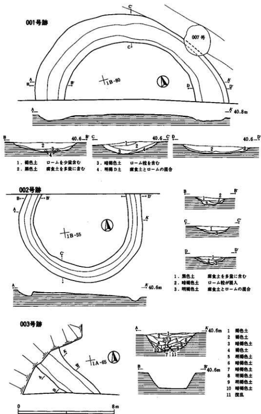
第4図 001・002・003号跡 (1/160・セクション1/80)
