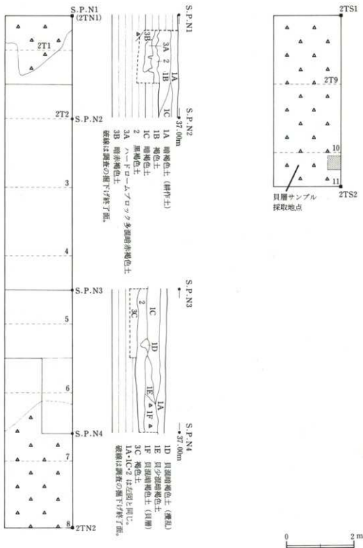
第4図 2T平面・土層断面図 (1/80)
