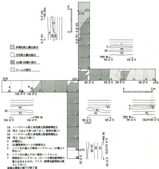
第6図 4T平面 (1/200)・土層断面図 (1/100)図
