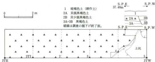
第5図 3T平面・土層断面図 (1/80)
