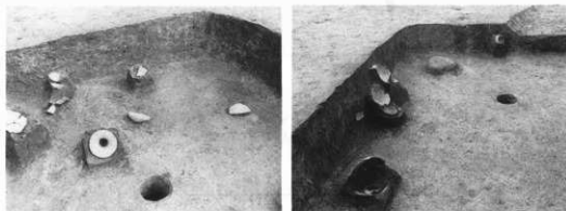
第10図 住居跡108遺物出土状況
