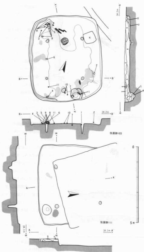
第7圖 住居跡103・111
