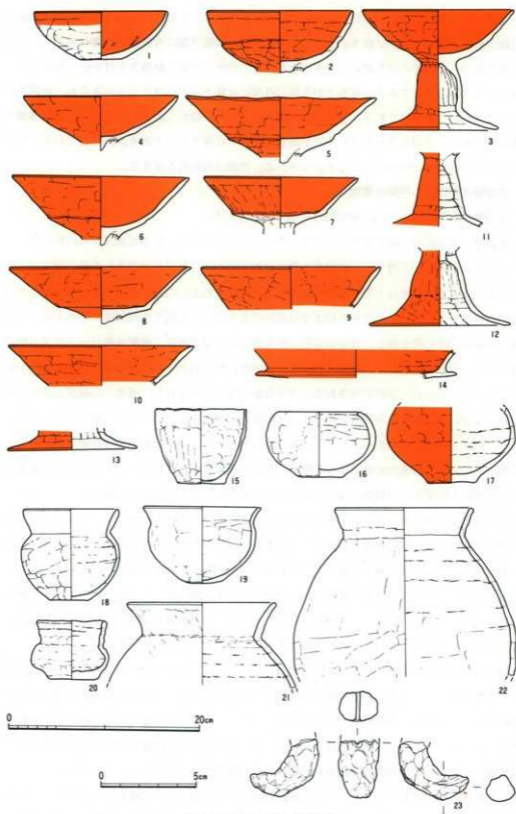
第32图 住居跡108出土遺物(1)
