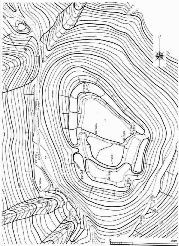
第31図 主郭遺構図 (S=1/500)
