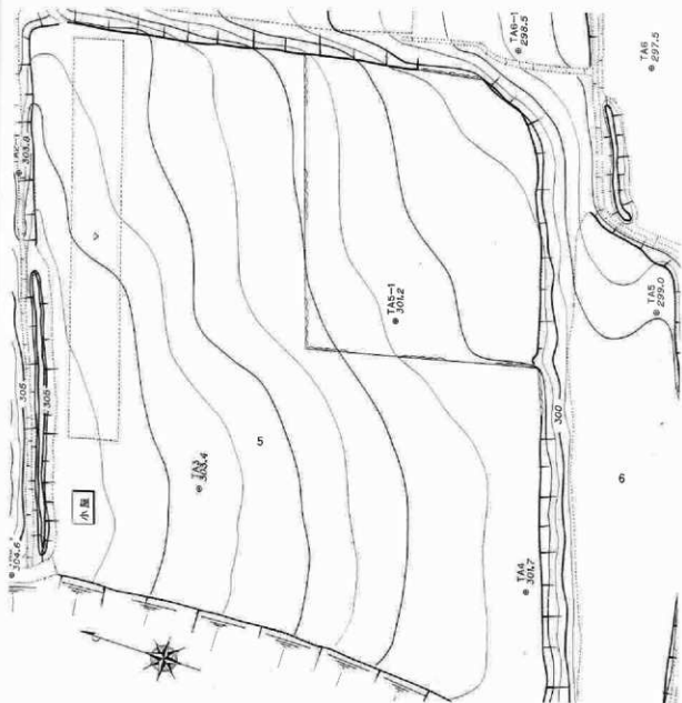
第25図 多賀氏屋敷跡遺構図 (S=1/500)
