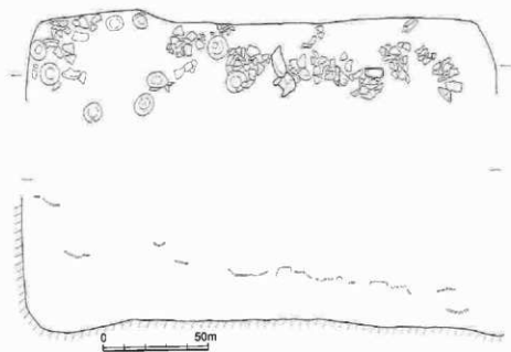
第46図 土師皿一括投棄遺構実測図
