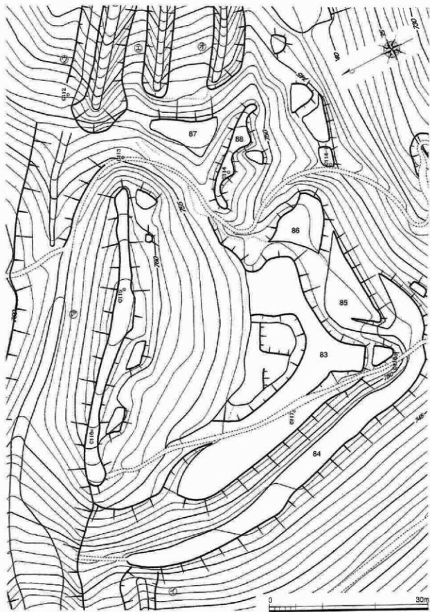
第40図 大堀切周辺遺構図 (S-1/500)
