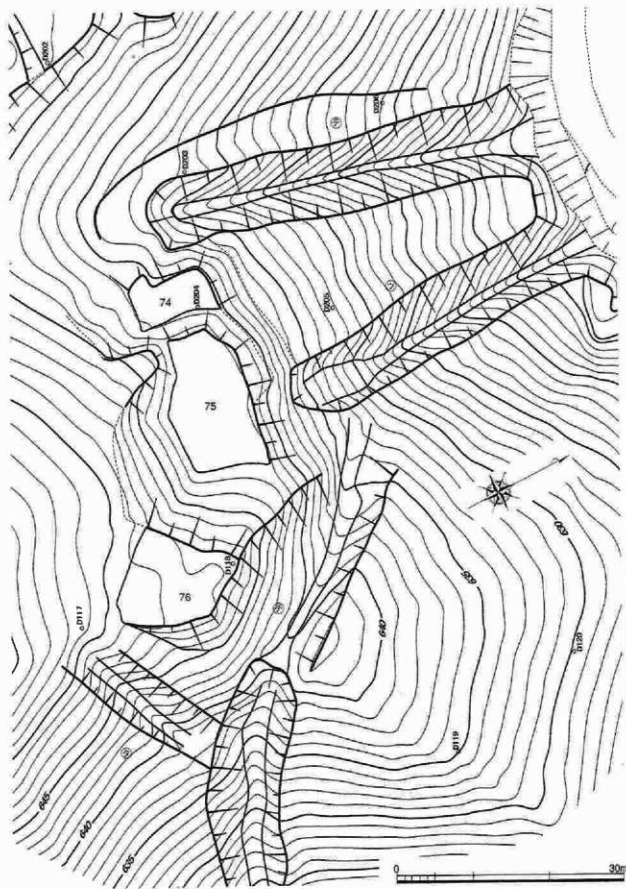
第41图 南西尾根部邊構圖
