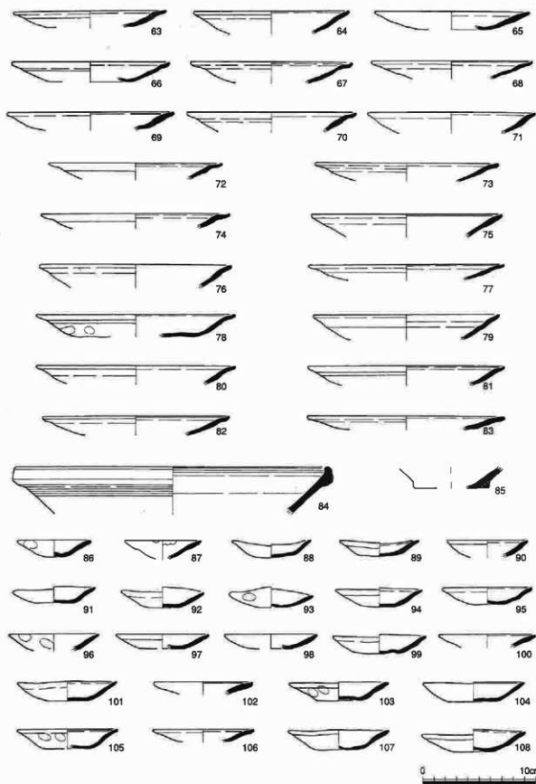
第48图 出土文物实测图(2)
