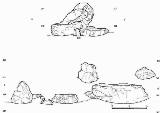
第19図 京極氏庭園跡景石立面図
