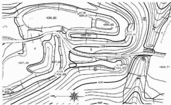
第32図 虎口遺構図 (S=1/500)
