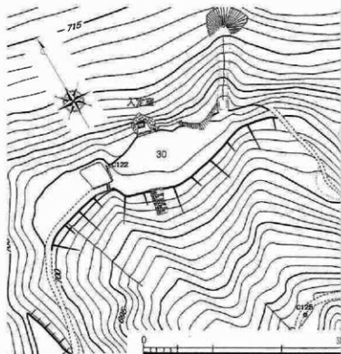
第38図 行者谷遺構図 (S=1/500)
