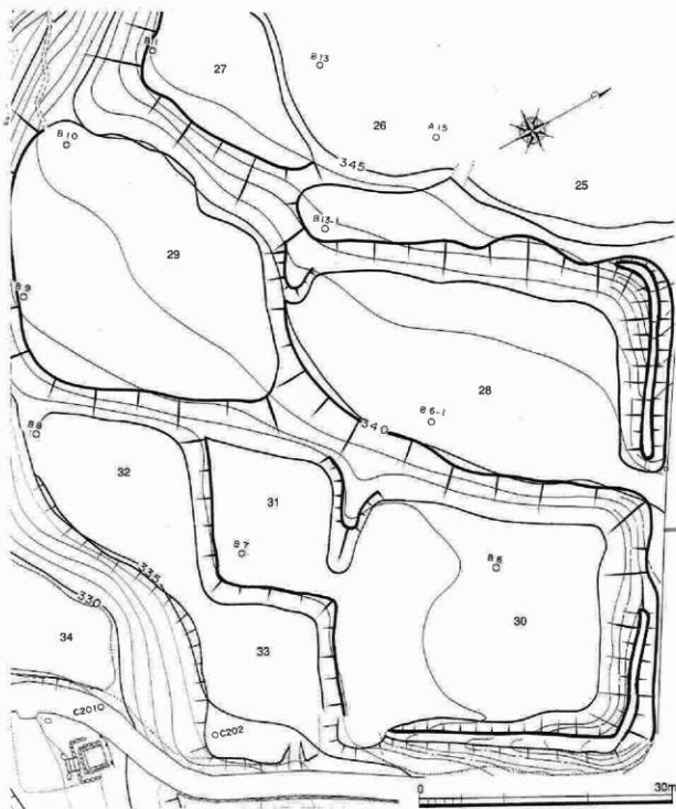
第17図 隠岐屋敷・畷跡遺構図 (S=1/500)
