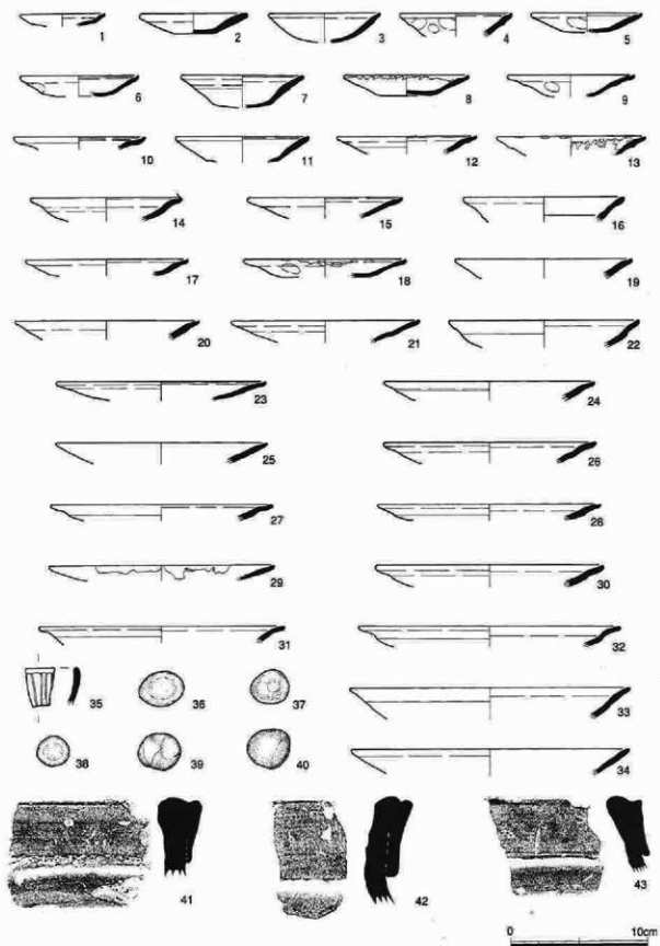
第43图 表探遺物実測図
