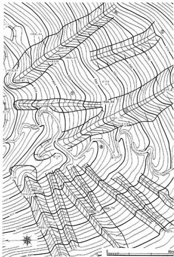
第33圖 壑場群遺構圖 (S=1/500)
