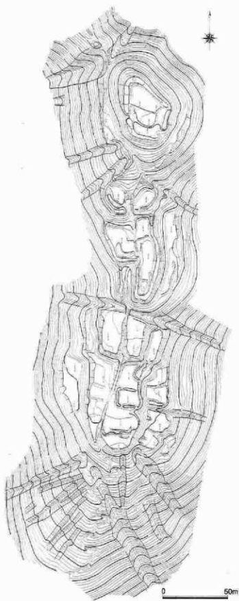
第29圖 上平寺城跡地形圖
