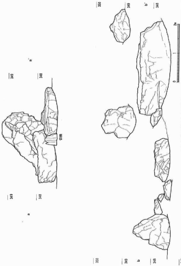
第4圖 京橋氏館跡埋蔵石立断面図
