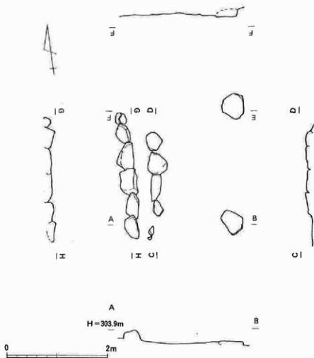
第4図 T2石列・礎石遺構実測図
