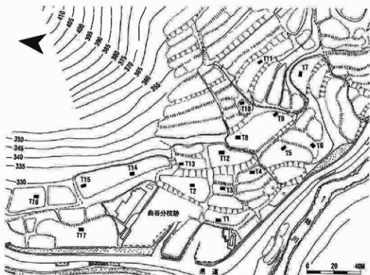
第6図 大平遺跡試堀トレンチ配置図
