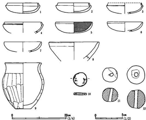
第26図 507号跡出土遺物実測図
