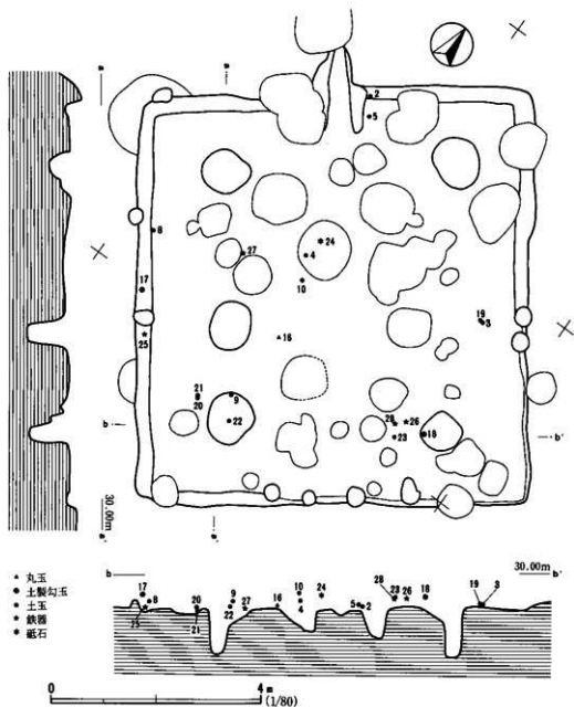
第22図 506号跡遺物出土状況
