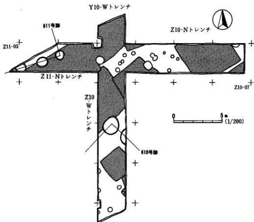
第16図 遺構確認状況図②
