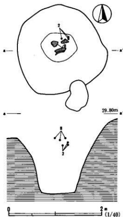
第12図 D501号跡実測図
