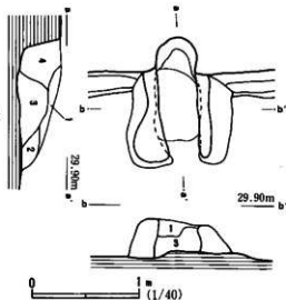
第9図 507号跡カマド実測図
