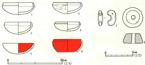
第19図 501号跡出土遺物実測図
