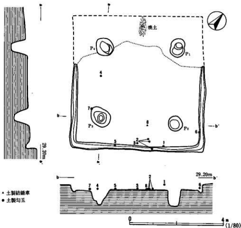
第5図 501号跡実測図
