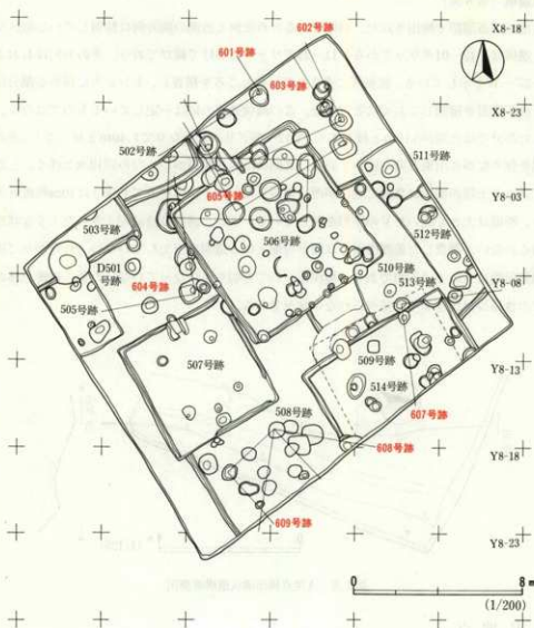
第7図 B地点遺構検出状況
