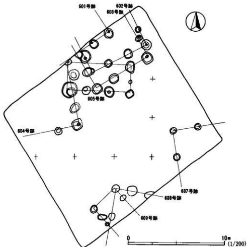
第10図 B地点掘立柱建物跡配置図
