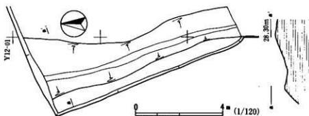
第6図 A地点検出溝状遺構実測図
