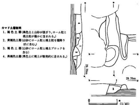
第8図 506号跡カマド実測図
