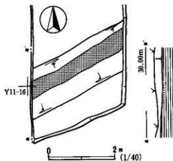
第15図 溝状遺構実測図
