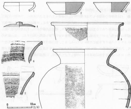
第34図 D501号跡出土遺物実測図
